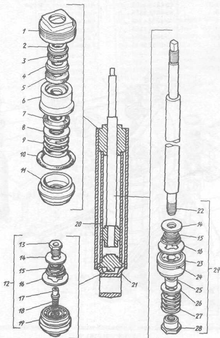
Рис. 34. Амортизаторы передние
