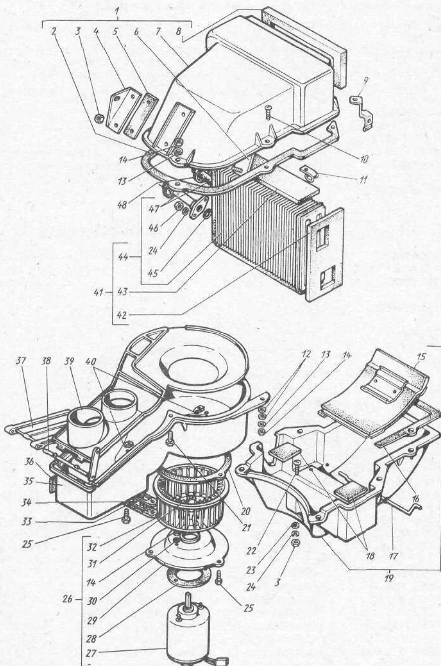
Рис. 88. Радиатор и электродвигатель отопителя
