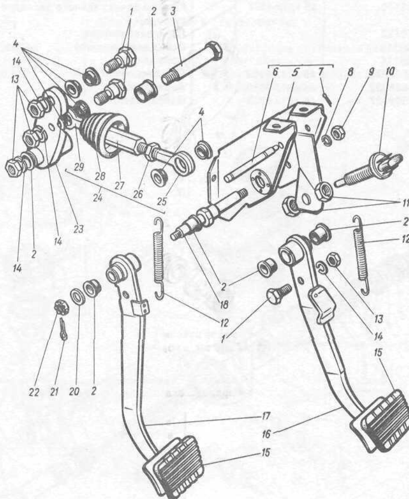
Рис. 47. Педаль сцепления и тормоза, привод механизма управления тормозами Примечания: 1. Поз. 2, 12, 15, 17, 20, 21, 22 см. в подгруппе 1602. 2. Поз. 10, 11 см. в подгруппе 3720.
