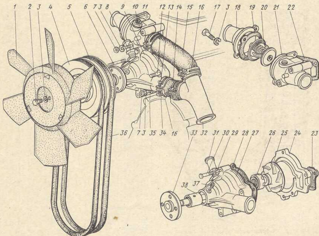
Рис. 20. Термостат, насос водяной, вентилятор и его привод Примечание. Поз. 10 см. в подгруппе 3828.
