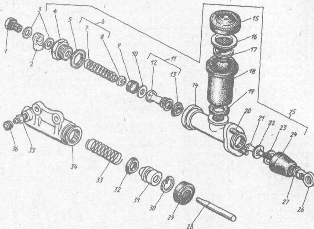
Рис. 22. Главный цилиндр привода сцепления и цилиндр выключения сцепления
