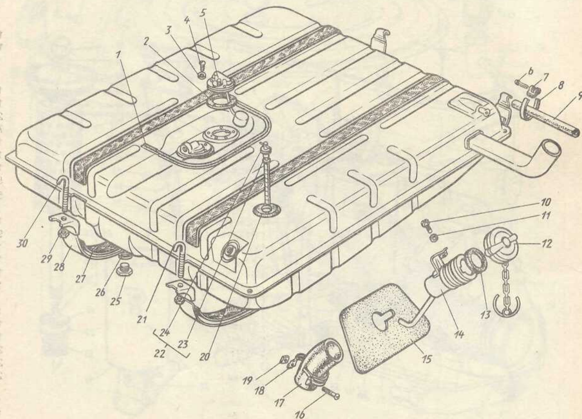
Рис. 10. Бак топливный
