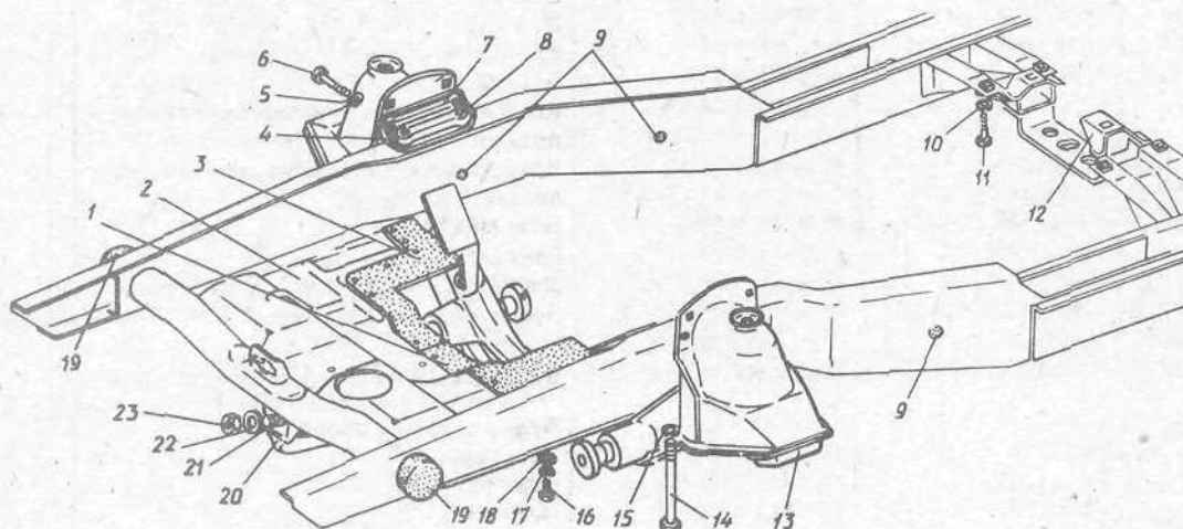
Рис. 29. Рама и брызговик двигателя
