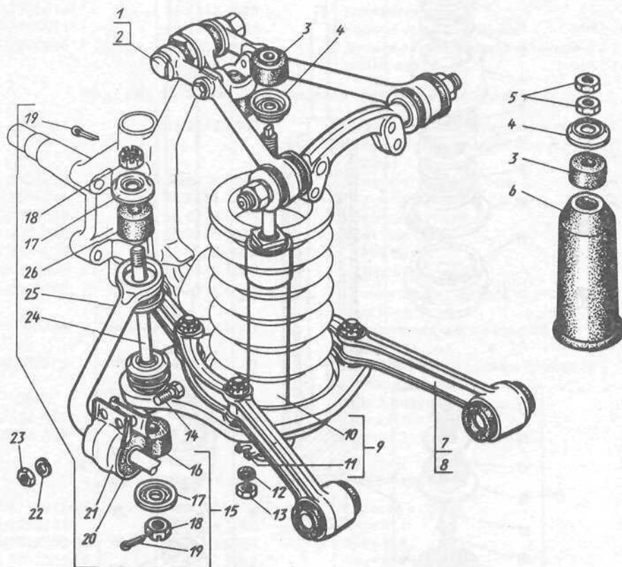
Рис. 33. Рычаги в сборе, амортизатор передней подвески и стабилизатор поперечной устойчивости
