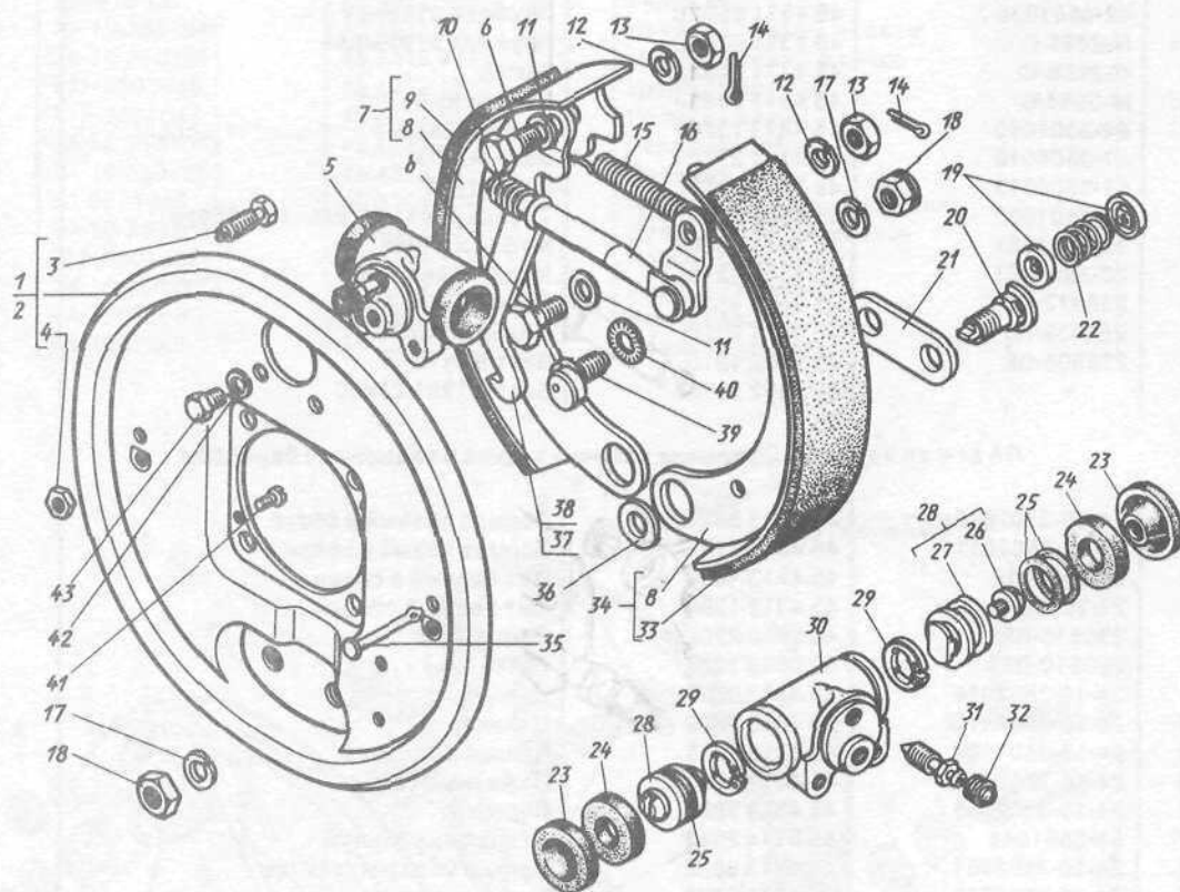
Рис. 46. Тормоза рабочие задние Примечание. Поз. 6, 10...14, 16...18, 37...40 см. в подгруппе 3508.
