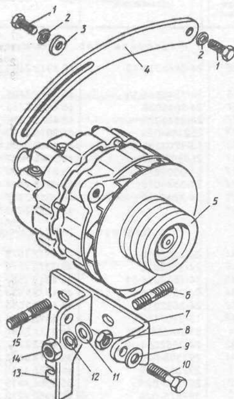
Рис. 53. Генератор
