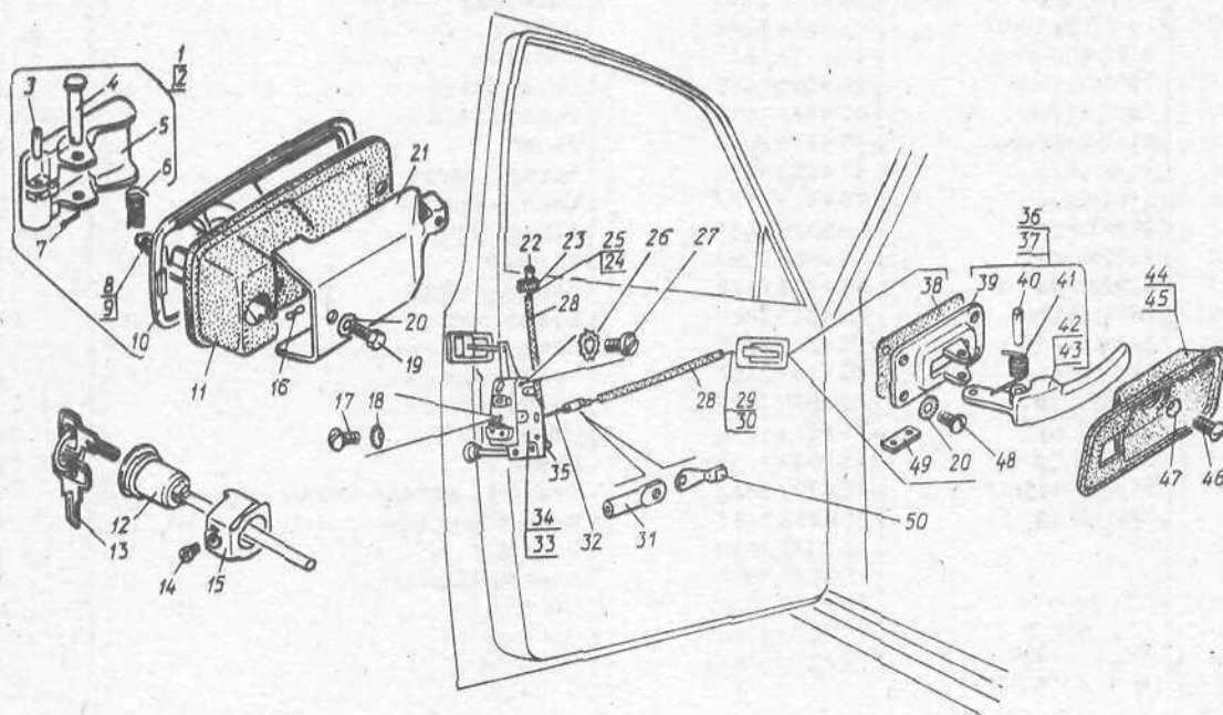
Рис. 81. Замок и ручки передней двери
