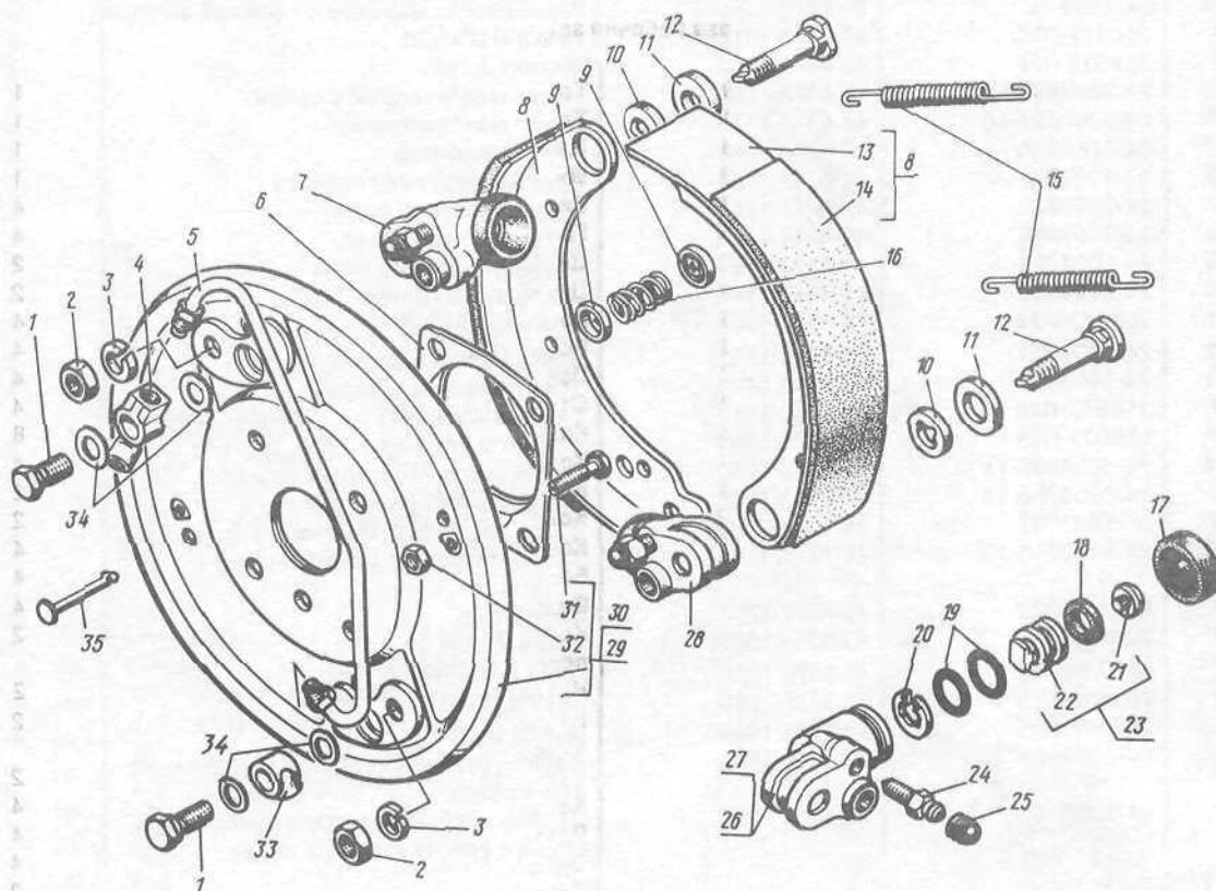
Рис. 45. Тормоза рабочие передние
