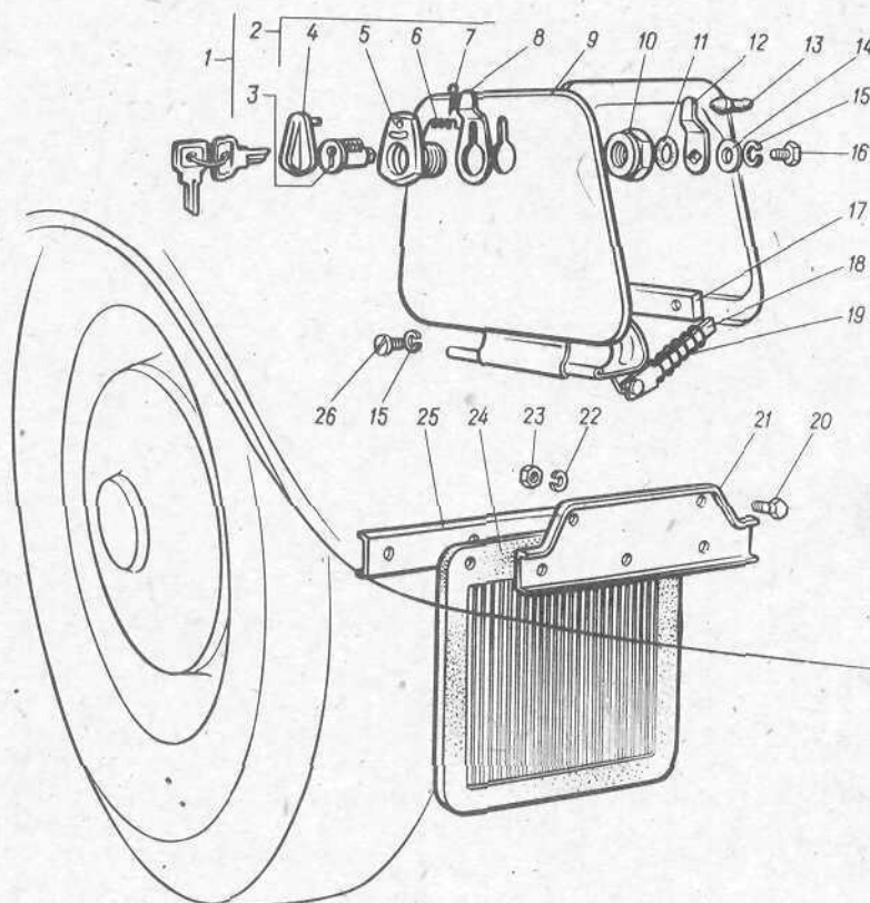
Рис. 96. Фартук щитка, люк заднего крыла
