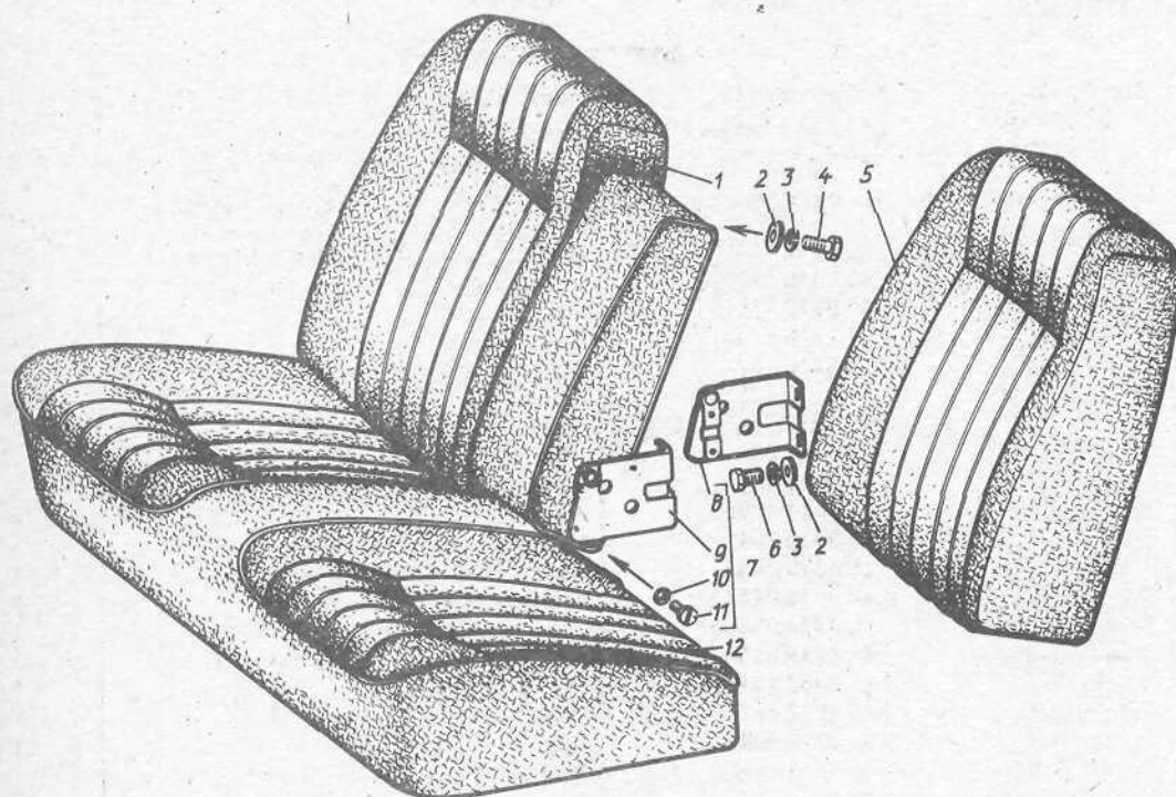
Рис. 86. Сиденье заднее
