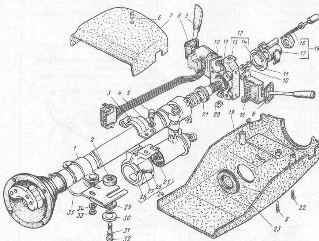
Рис. 42. Управление рулевое
