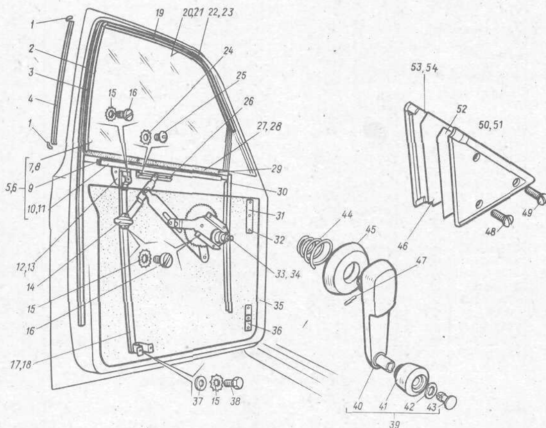
Рис. 80. Окно и механизм перемещения стекла передней двери
