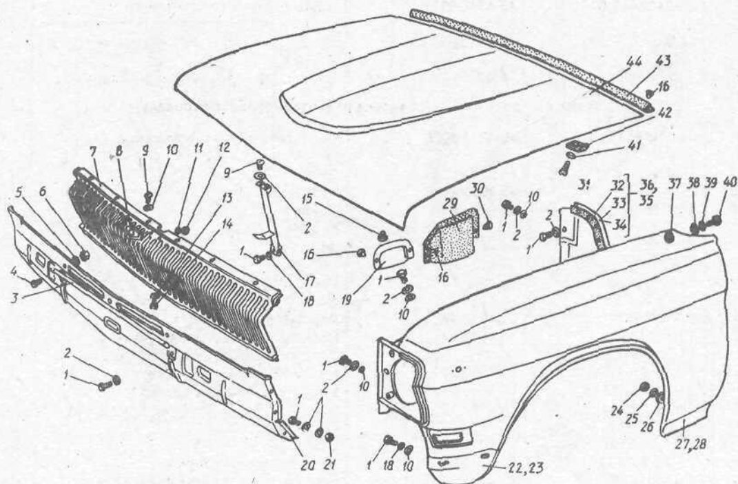
Рис. 94. Облицовка радиатора (металлическая), капот, крыло переднее
