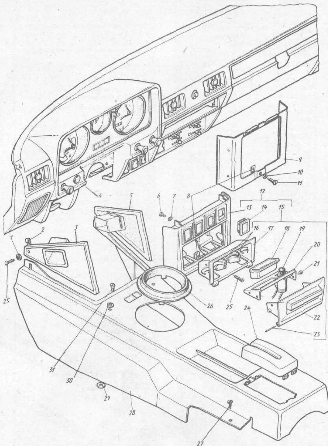
Рис. 116. Панель приборов, консоль панели приборов, пепельница
