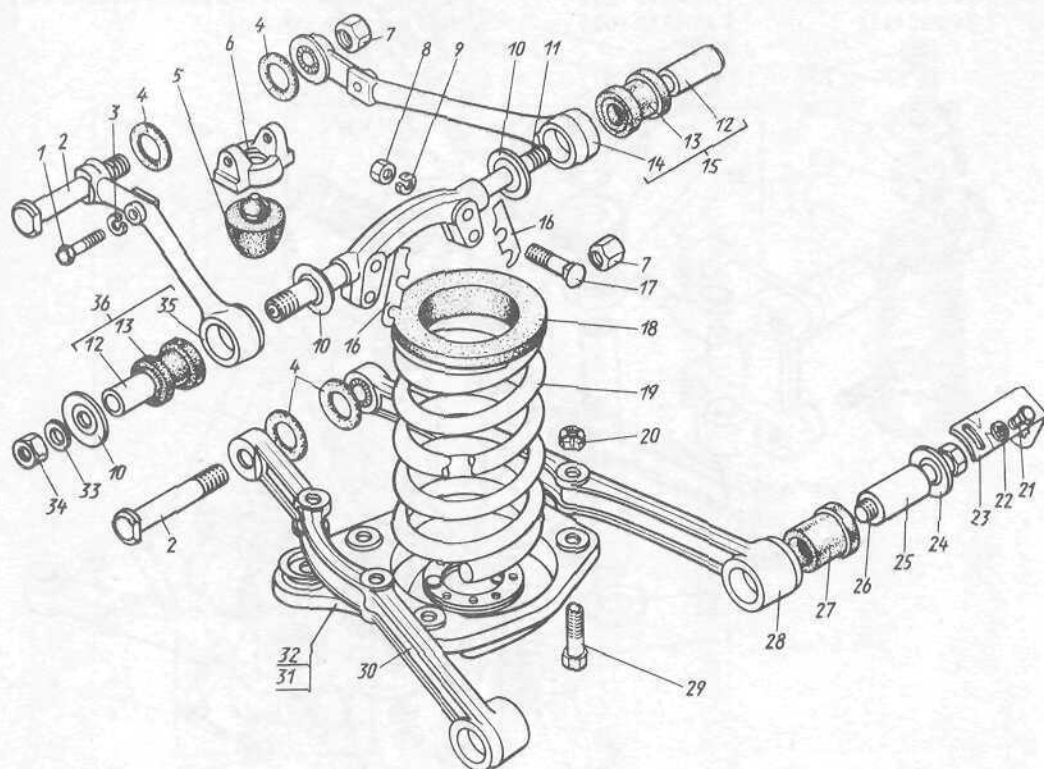
Рис. 31. Пружины и рычаги передней подвески
