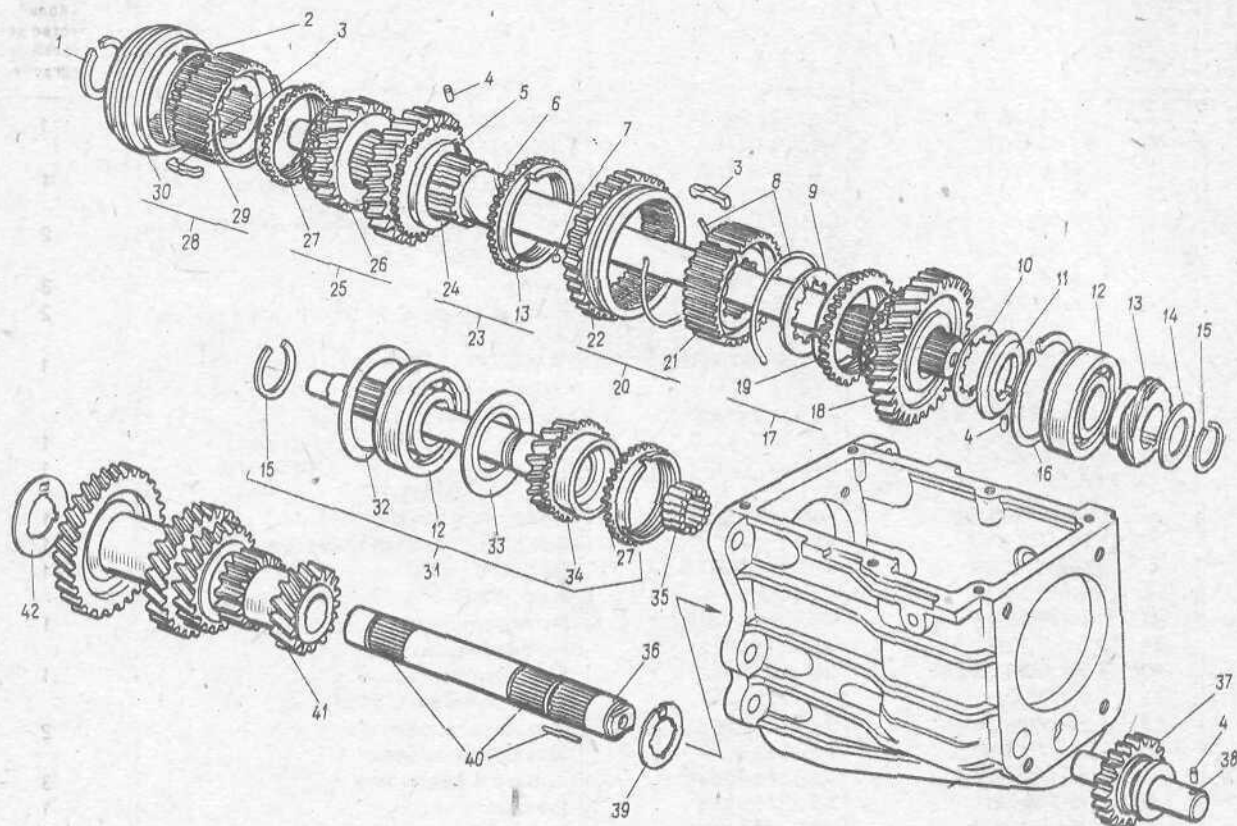
Рис. 24. Коробка передач
