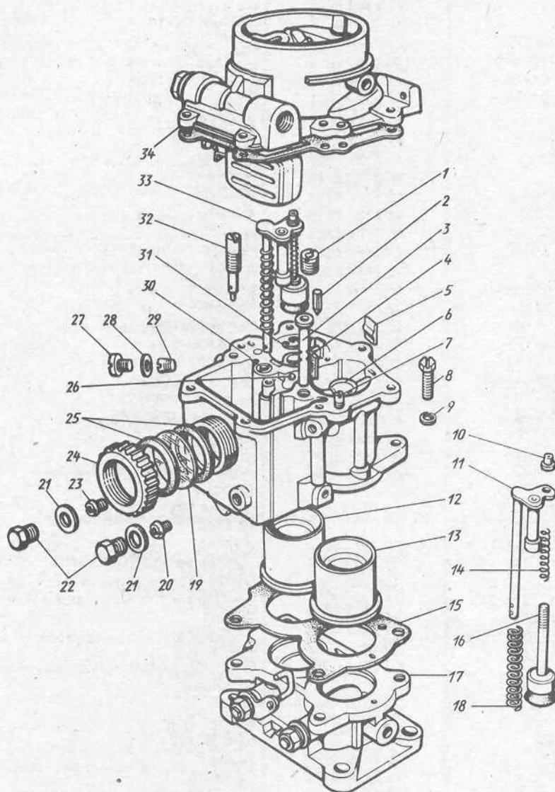
Рис. 107. Карбюратор
