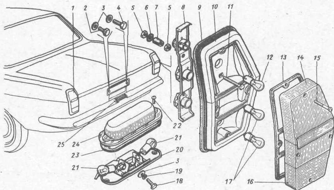
Рис. 61. Фонари задние, фонарь освещения номерного знака
