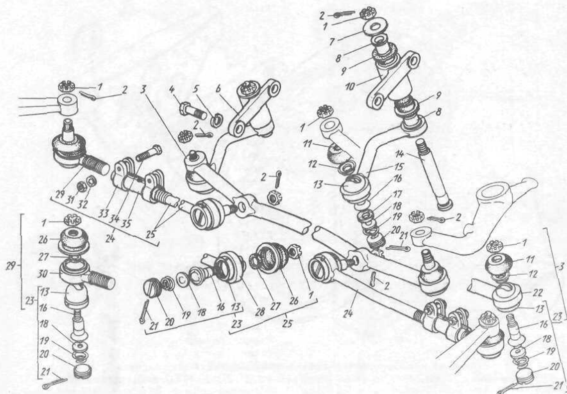
Рис. 44. Тяги рулевые
