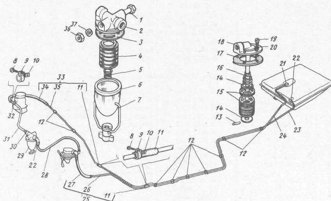
Рис. 105. Трубопроводы топливные и фильтр тонкой очистки топлива. Примечание: Поз. 1...7, 29, 36, 37 см. в подгруппе 1117.
