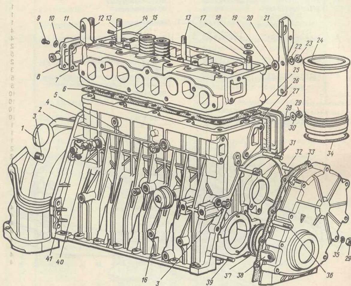
Рис. 3. Блок и головка цилиндров двигателя
