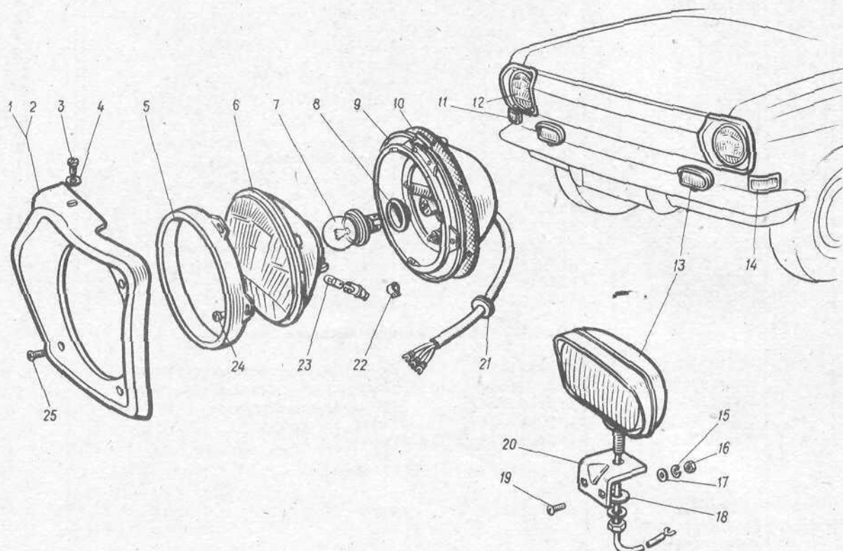
Рис. 59. Фары, указатели поворота и фары противотуманные Примечания: 1. Поз. 11, 14 см. в подгруппе 3726. 2. Поз. 13, 15...20 см. в подгруппе 3743.
