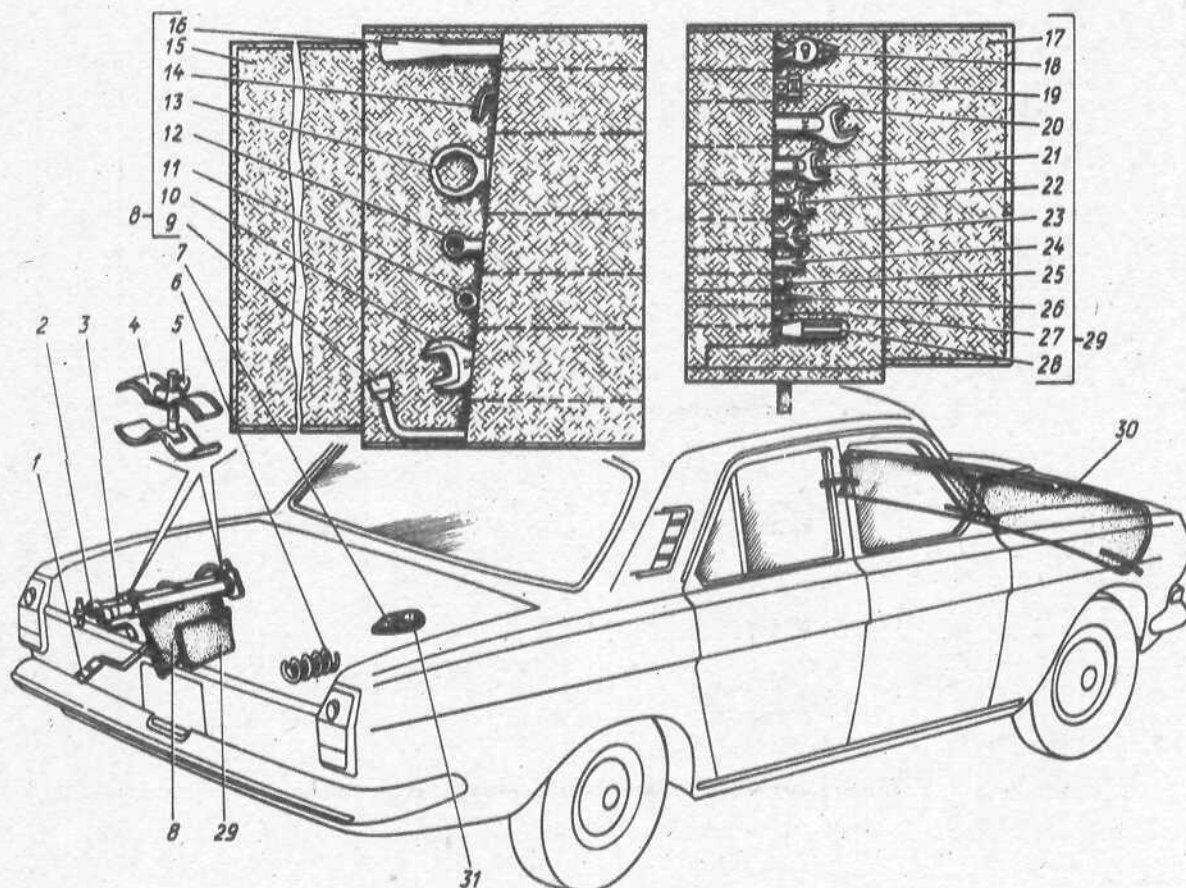
Рис. 67. Инструмент водителя и приспособления
