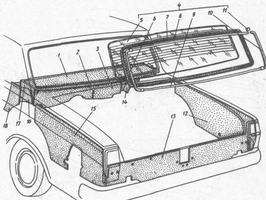
Рис. 77. Обивка полки задка, окно задка, обивка багажника Примечание. Поз. 3, 12, 13, 15 см. в подгруппе 5608.
