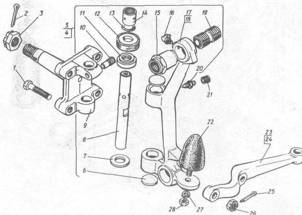
Рис. 32. Стойки передней подвески и поворотные кулаки
