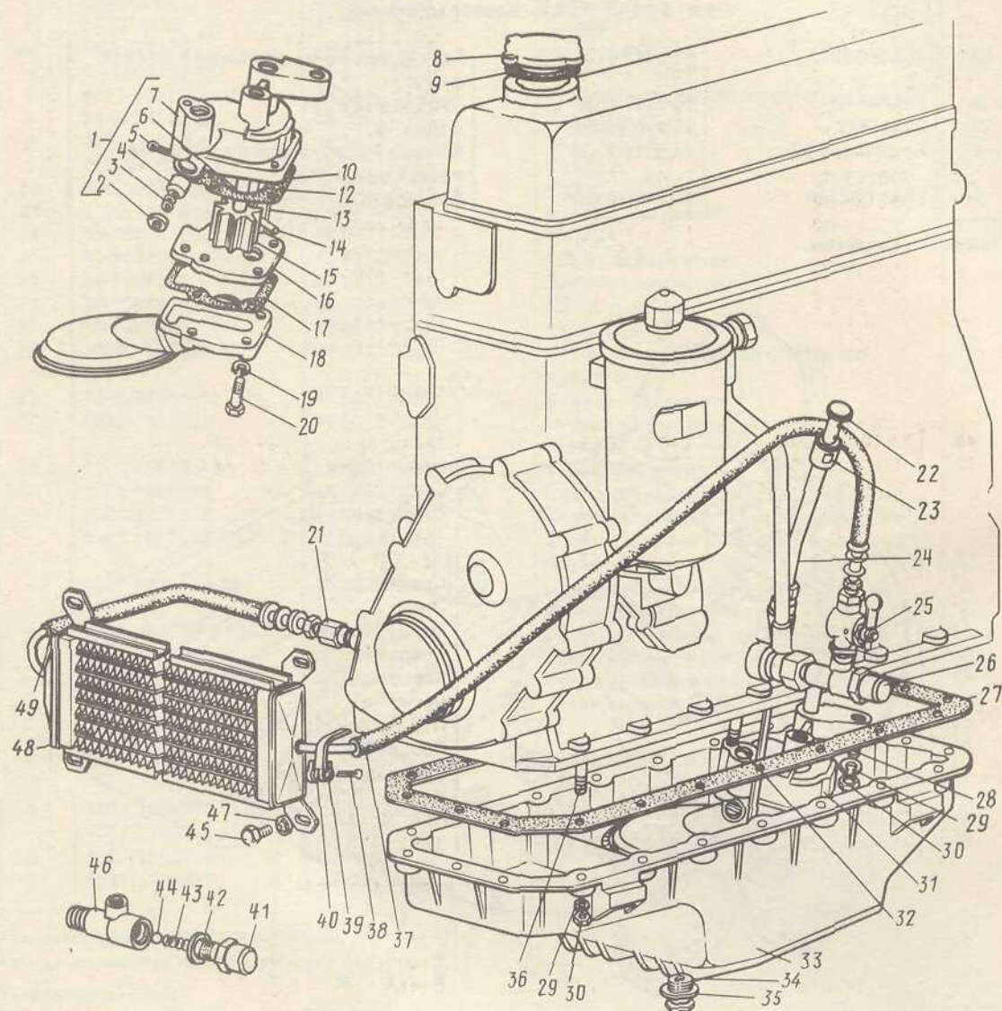
рис. 7. Картер масляный, насос масляный и радиатор масляный
