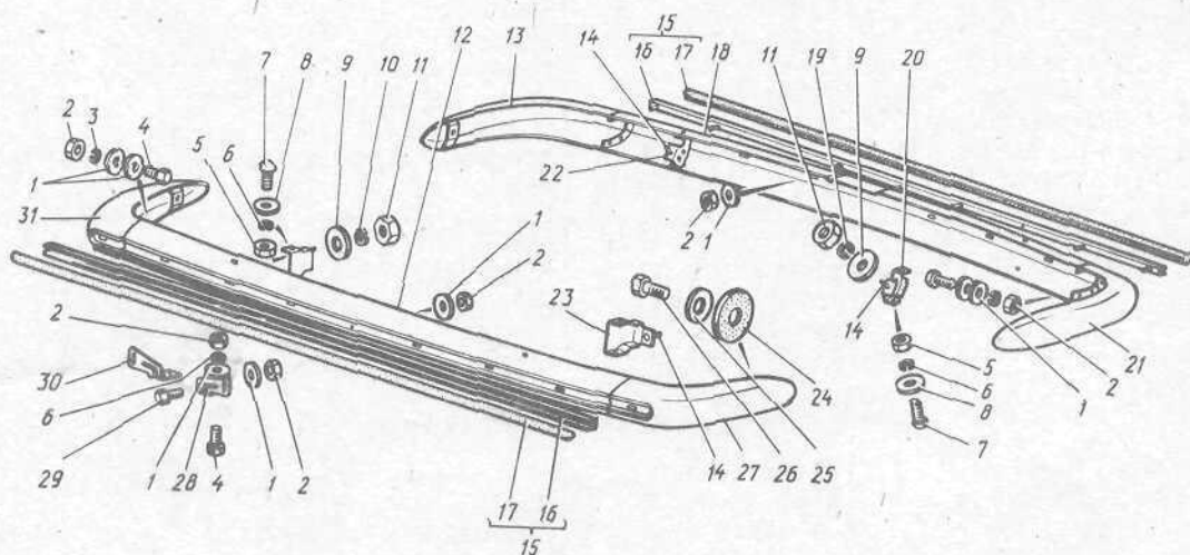
Рис. 30. Буфер передний и задний
