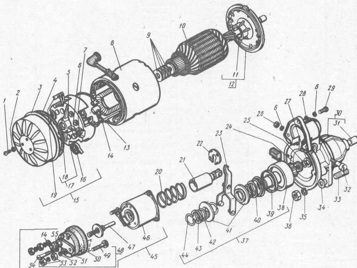
Рис. 58. Стартер
