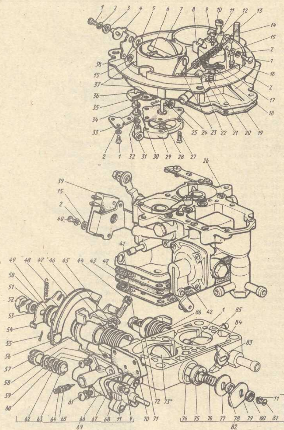
Рис. 13. Карбюратор
