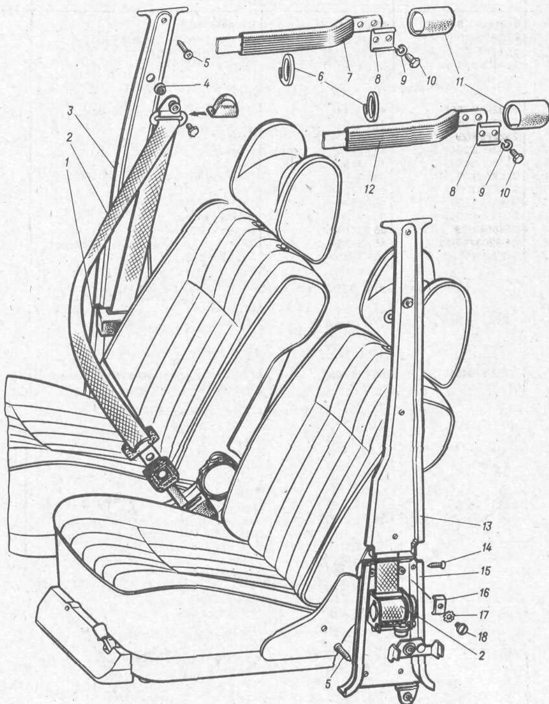
Рис. 92. Держатели, поручни, крючки для одежды, ремни безопасности Примечания: 1. Поз. 3, 5, 13, 14 см. в подгруппе 5401. 2. Поз. 1, 2, 4, 5, 14...18 см. в подгруппе 8217.
