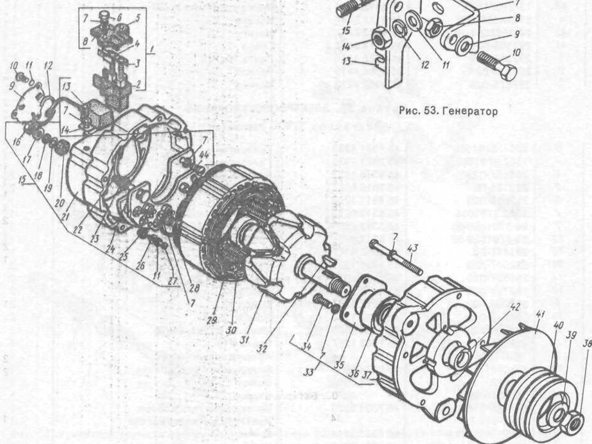
Рис. 54. Генератор
