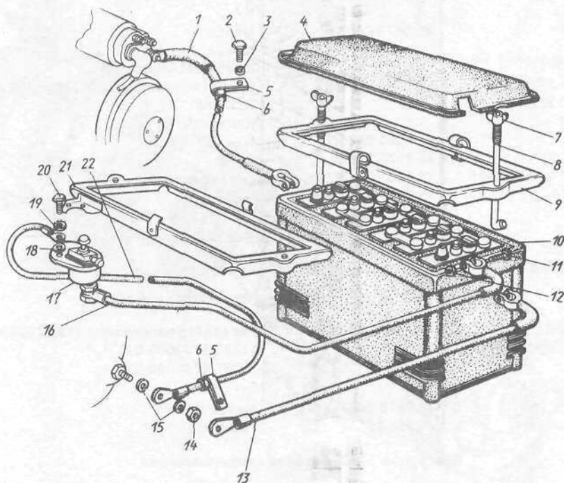
Рис. 55. Батарея аккумуляторная
