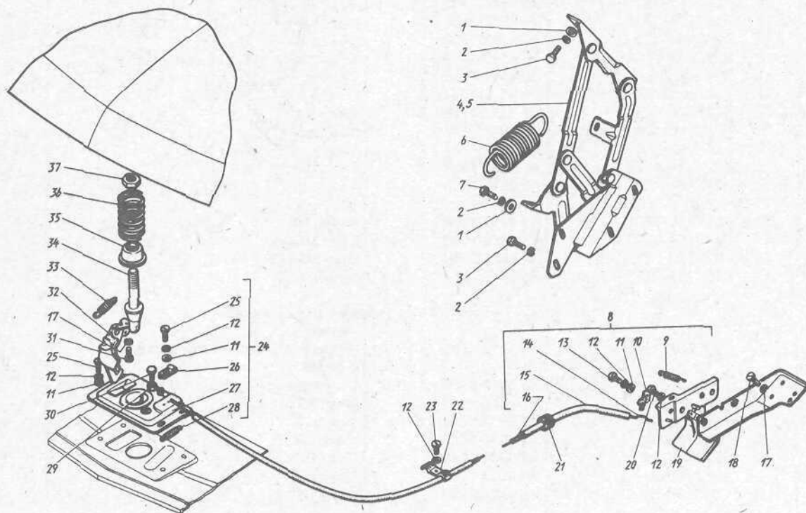
Рис. 97. Замок и привод замка капота, петли капота
