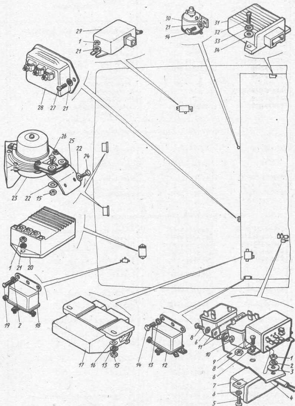
Рис. 62. Электрооборудование
