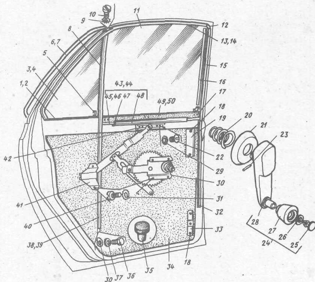
Рис. 83. Окно и механизм перемещения стекла задней двери
