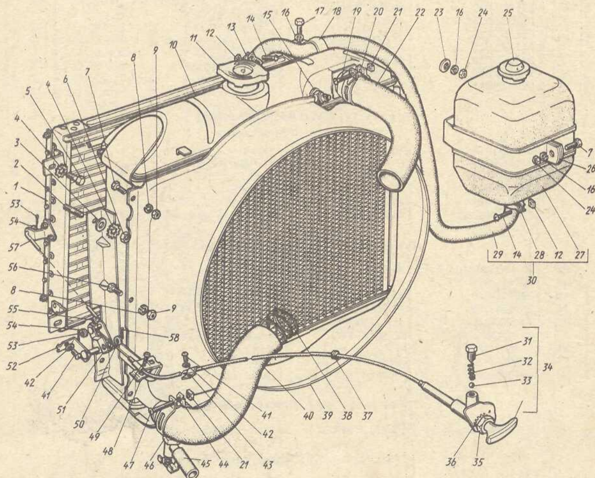
Рис. 19. Радиатор, трубопроводы и шланги, пробка радиатора, краник сливной, кожух вентилятора, жалюзи и расширительный бачок
