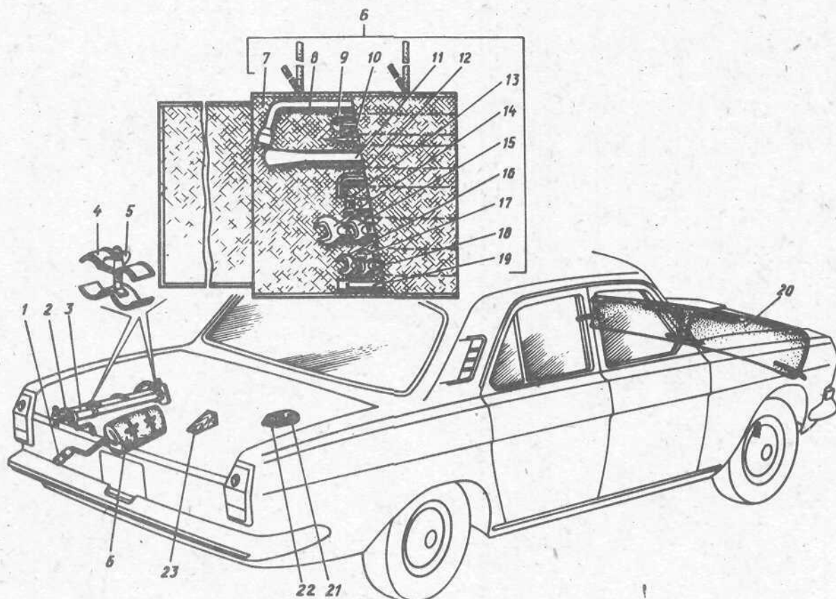
Рис. 68. Инструмент водителя и приспособления (для экспорта)
