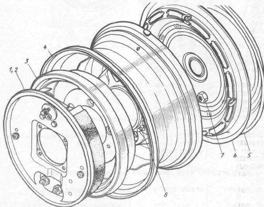
Рис. 37. Колеса, колпаки колес, тормоза рабочие задние в сборе и тормозные барабаны
