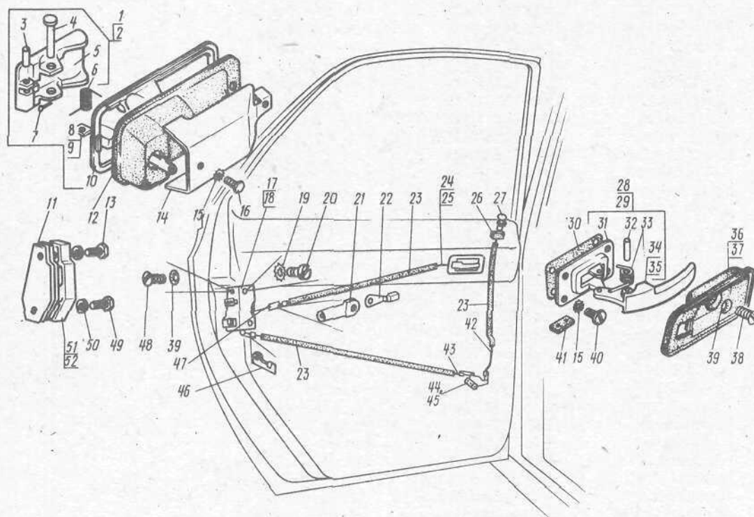
Рис. 84. Замок и ручки задней двери
