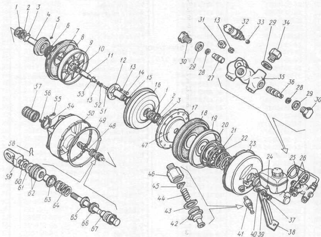
Рис. 52. Усилитель тормоза вакуумный, сигнализация прекращения действия тормозов аварийная, трубопроводы вакуумного усилителя тормоза.
