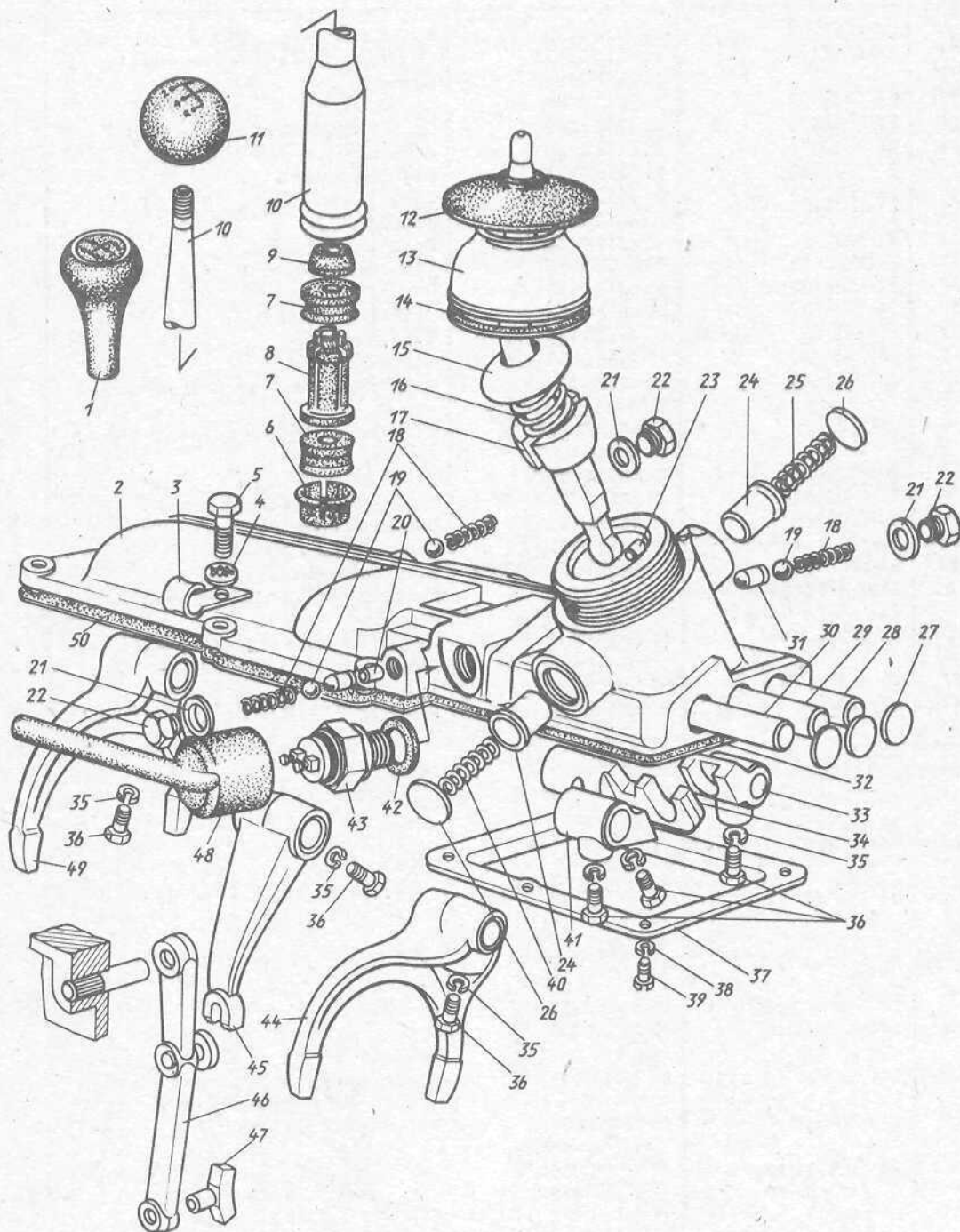
Рис. 26. Механизм переключения передач
