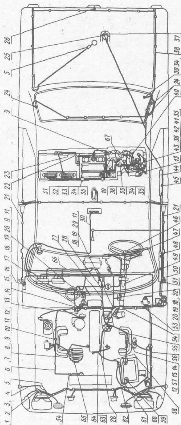
Рис. 64. Соединители электропроводов, электропровода (для модели ГАЗ-24-11) Примечания: 1. Поз. 28 см. в подгруппе 3707. 2. Поз. 1, 2, 3, 52 см. в подгруппе 3723.
