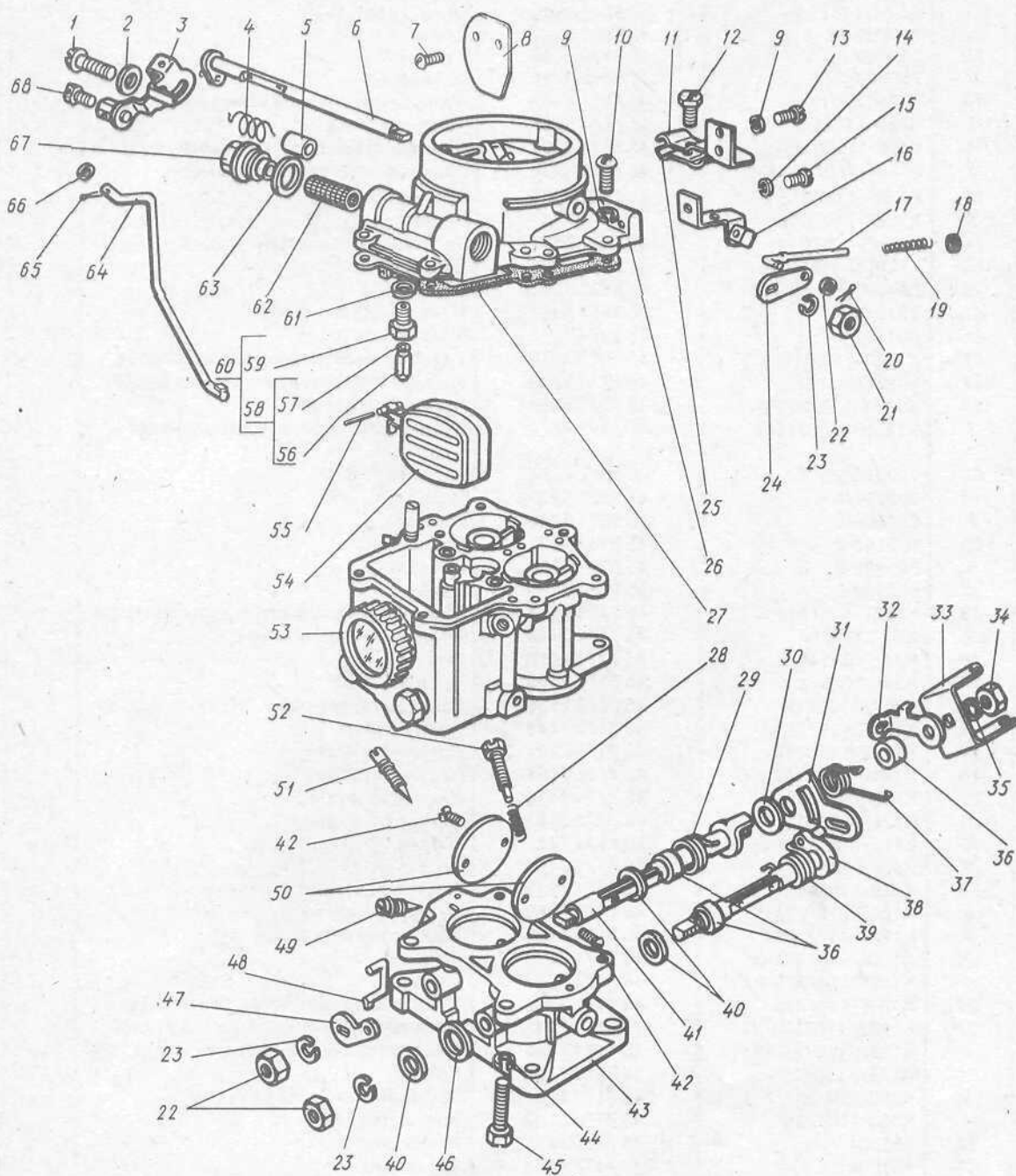
Рис. 106. Карбюратор
