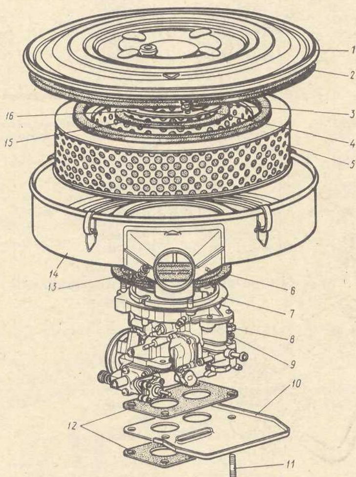
Рис. 16. Фильтр воздушный и установка карбюратора
