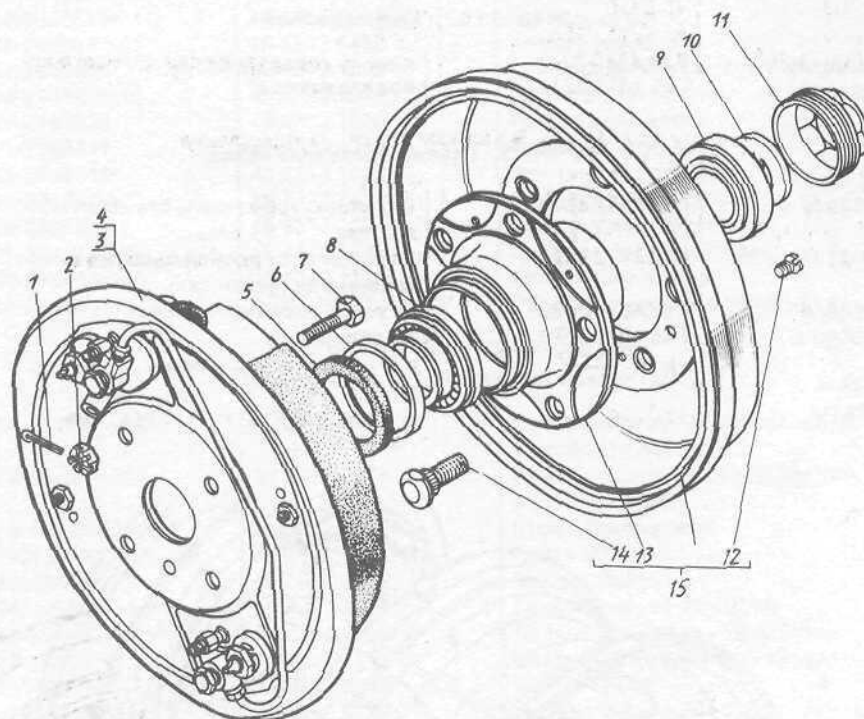
Рис. 38. Ступицы передних колес, тормоза рабочие передние Примечание. Поз. 1...4, 7, 12 см. в подгруппе 3501.
