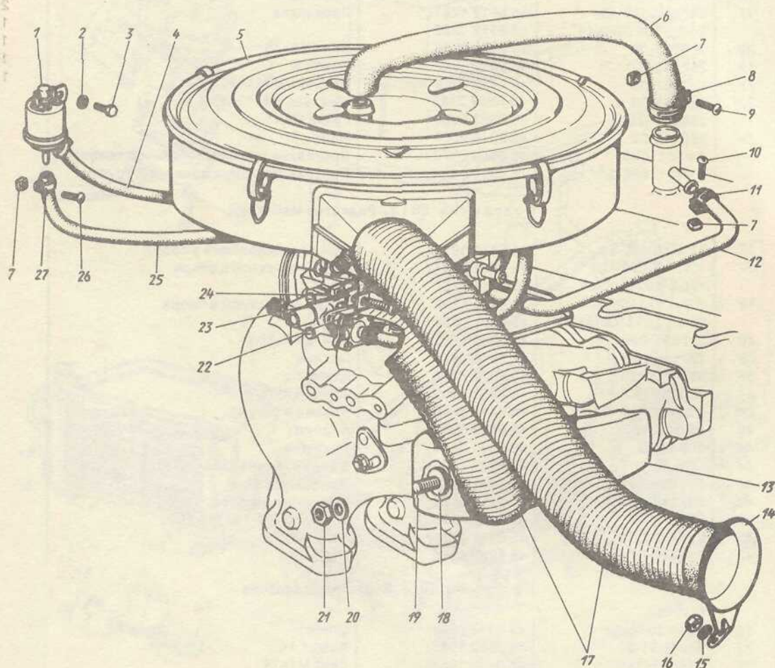
Рис. 8. Вентилиция картера, фильтр воздушный двигателя и устройства дополнительные карбюратора Примечания: 1. Поз. 5, 13... 24 см. в подгруппе 1109. 2. Поз. 1...4, 25...27 см. в подгруппе 1127.
