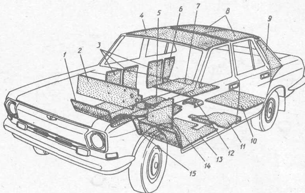
Рис. 71. Термошумоизоляция кузова
