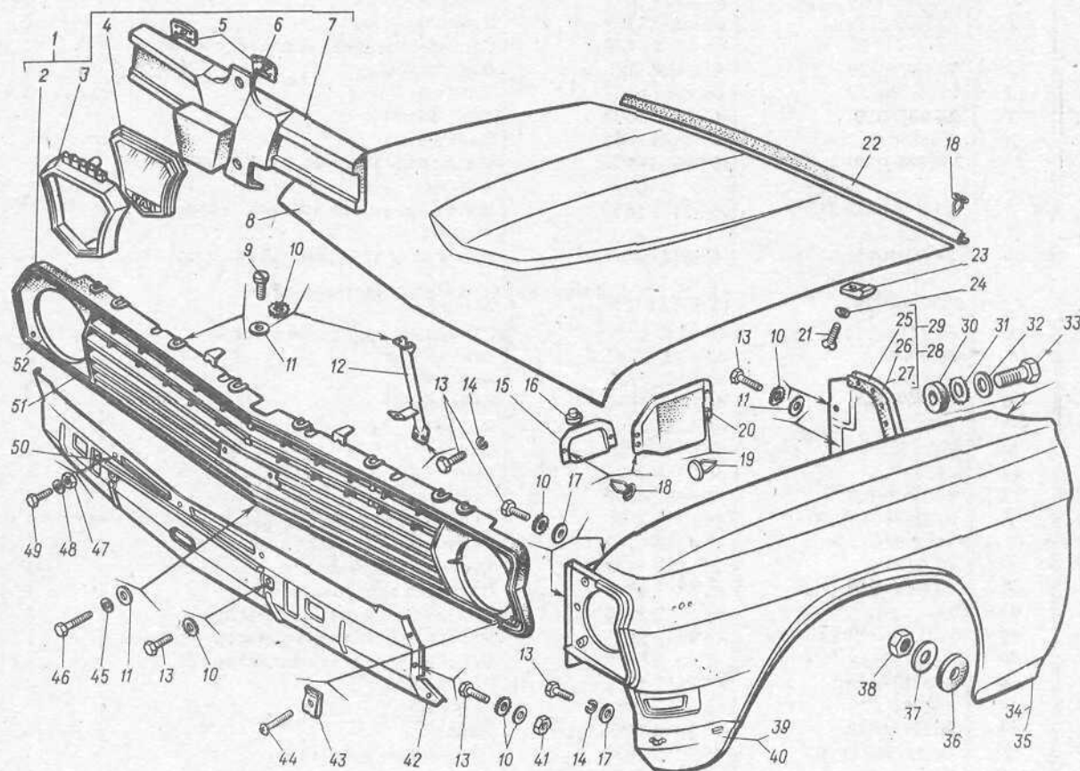
Рис. 95. Облицовка радиатора (пластмассовая), капот, крыло переднее
