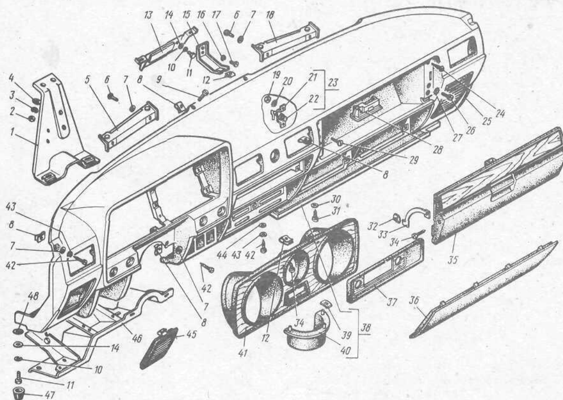
Рис. 74. Панель приборов и вещевого ящик
