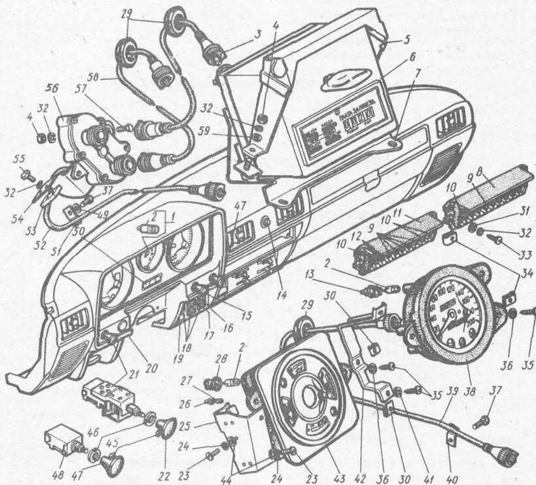
Рис. 66. Панель и комбинация приборов
