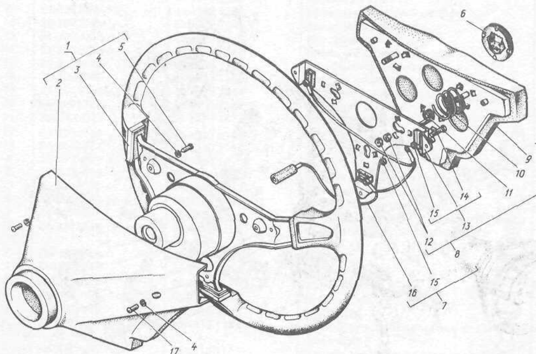
Рис. 43. Колесо рулевого управления и кнопка звукового сигнала
