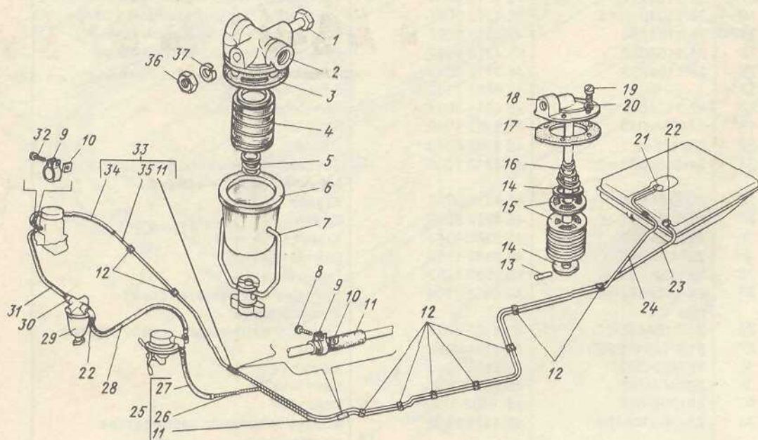
Рис. 11. Трубопроводы топливные и фильтр тонкой очистки топлива
