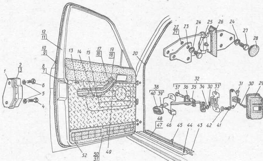
Рис. 79. Дверь передняя
