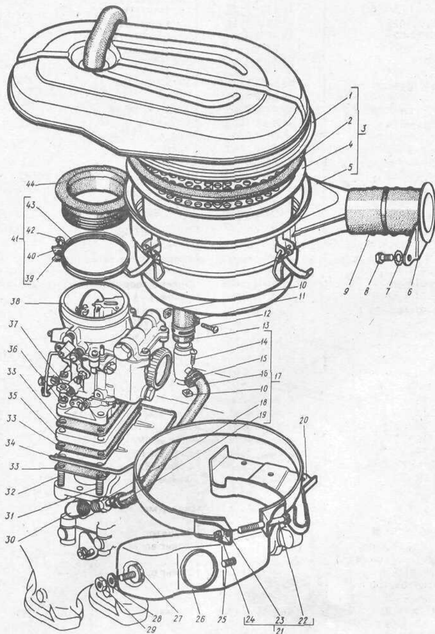
Рис. 103. Вентилиция картера, карбюратор и фильтр воздушный двигателя Примечания: 1. Поз. 31...38 см. в подгруппе 1107. 2. Поз. 1...9, 20...29, 39...44 см. в подгруппе 1109.
