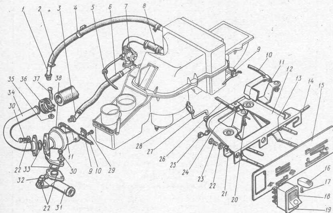
Рис. 90. Управление вентиляцией и отоплением кузова, трубопроводы
