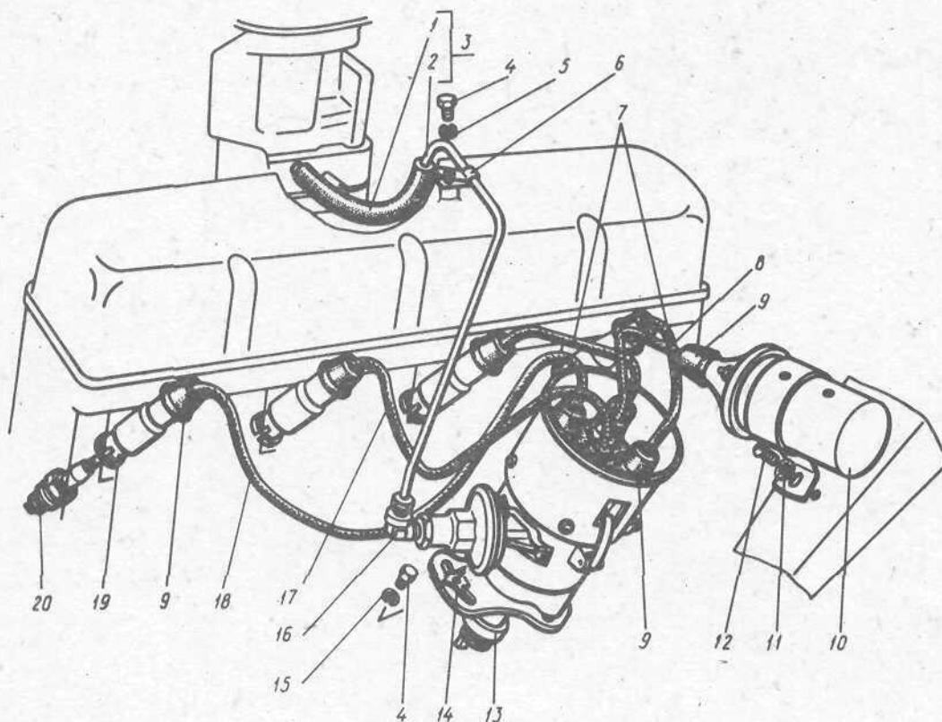
Рис. 56. Катушка зажигания, датчик-распределитель, свечи и провода зажигания
