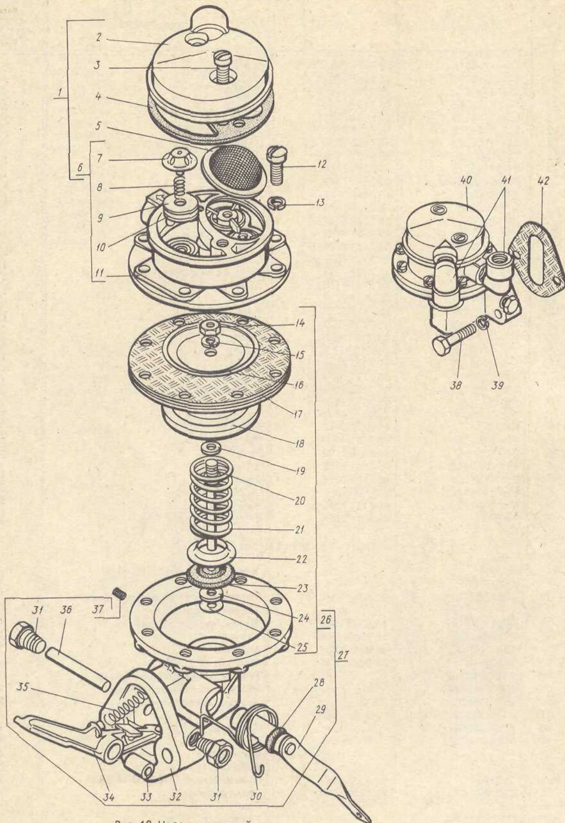
Рис. 12. Насос топливный
