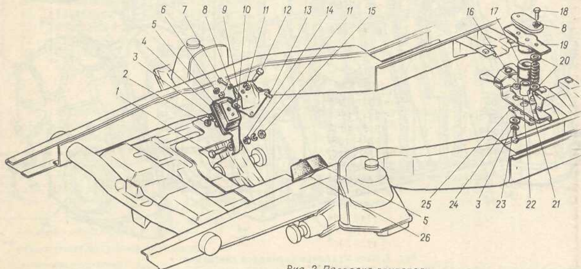
Рис. 2. Подвеска двигателя
