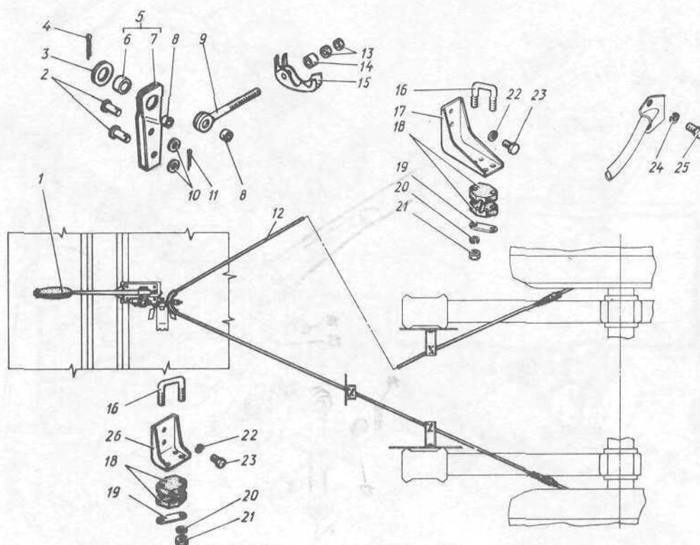
Рис. 50. Привод механизма управления стояночным тормозом
