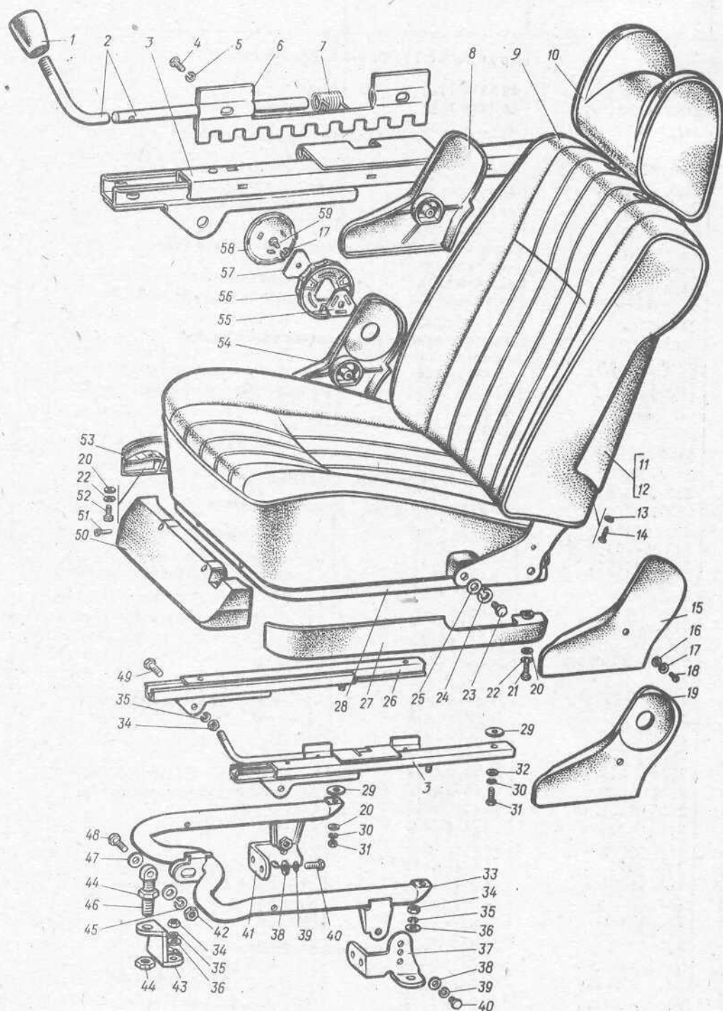
Рис. 85. Сиденье водителя и переднее сиденье
