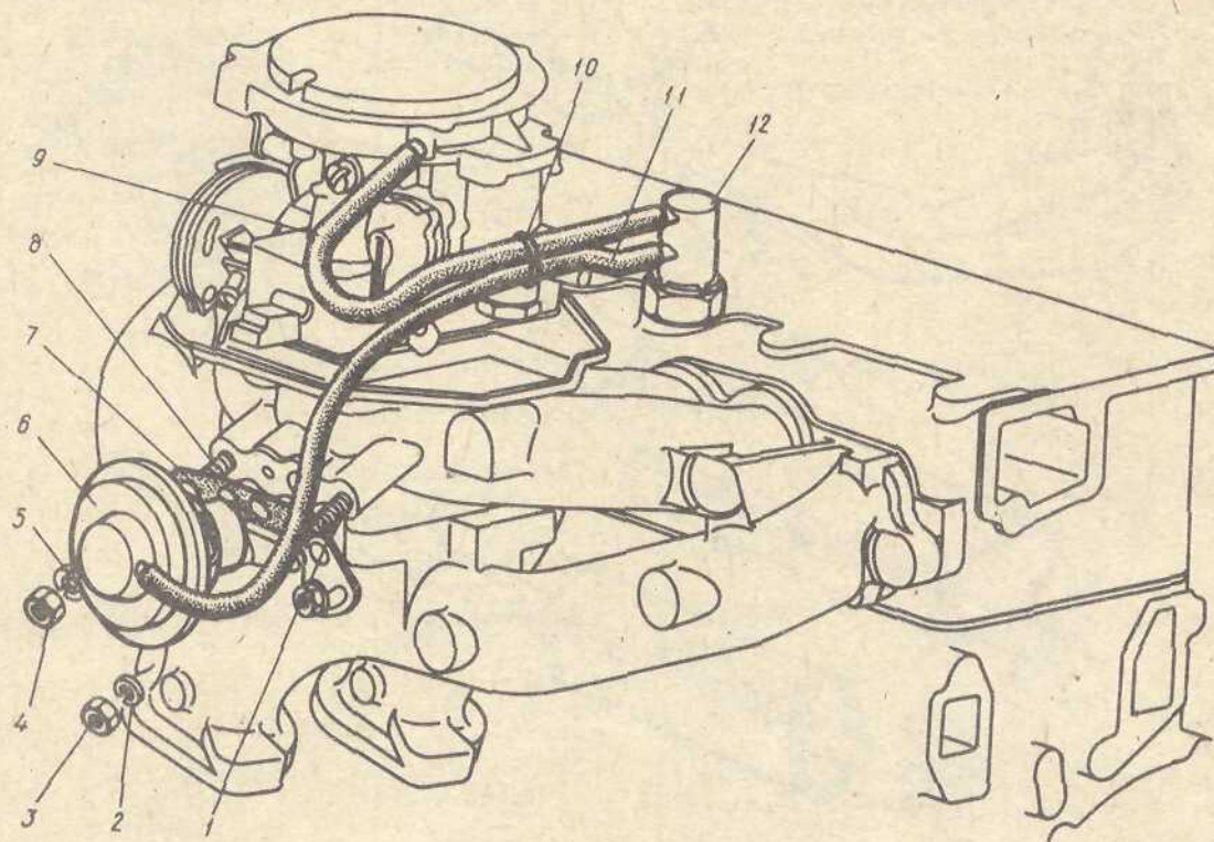
Рис. 18. Система рециркуляции отработавших газов
