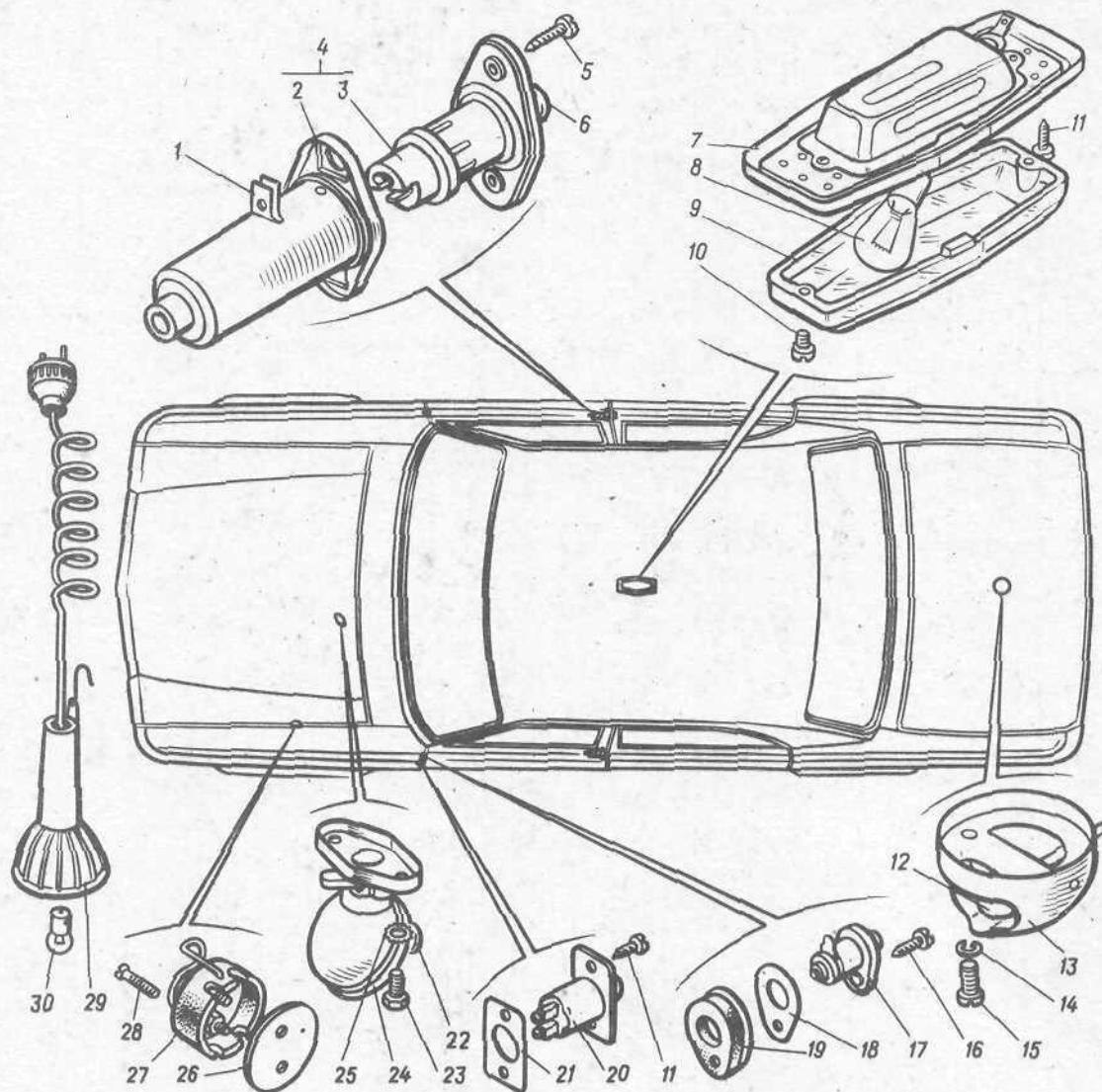
Рис. 60. Плафоны внутреннего освещения, лампы переносная и подкапотная
