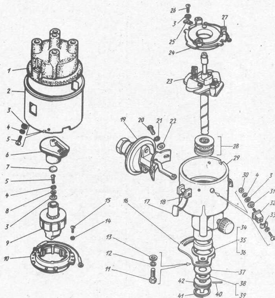
Рис. 57. Датчик-распределитель
