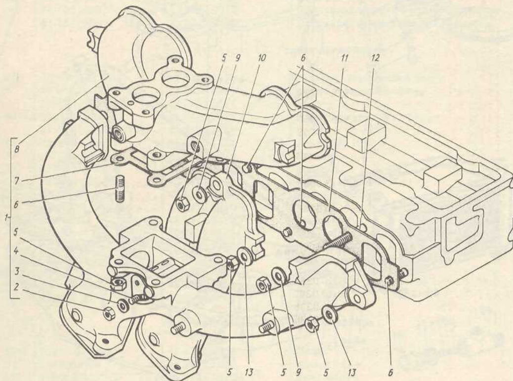
Рис. 6. Газопровод
