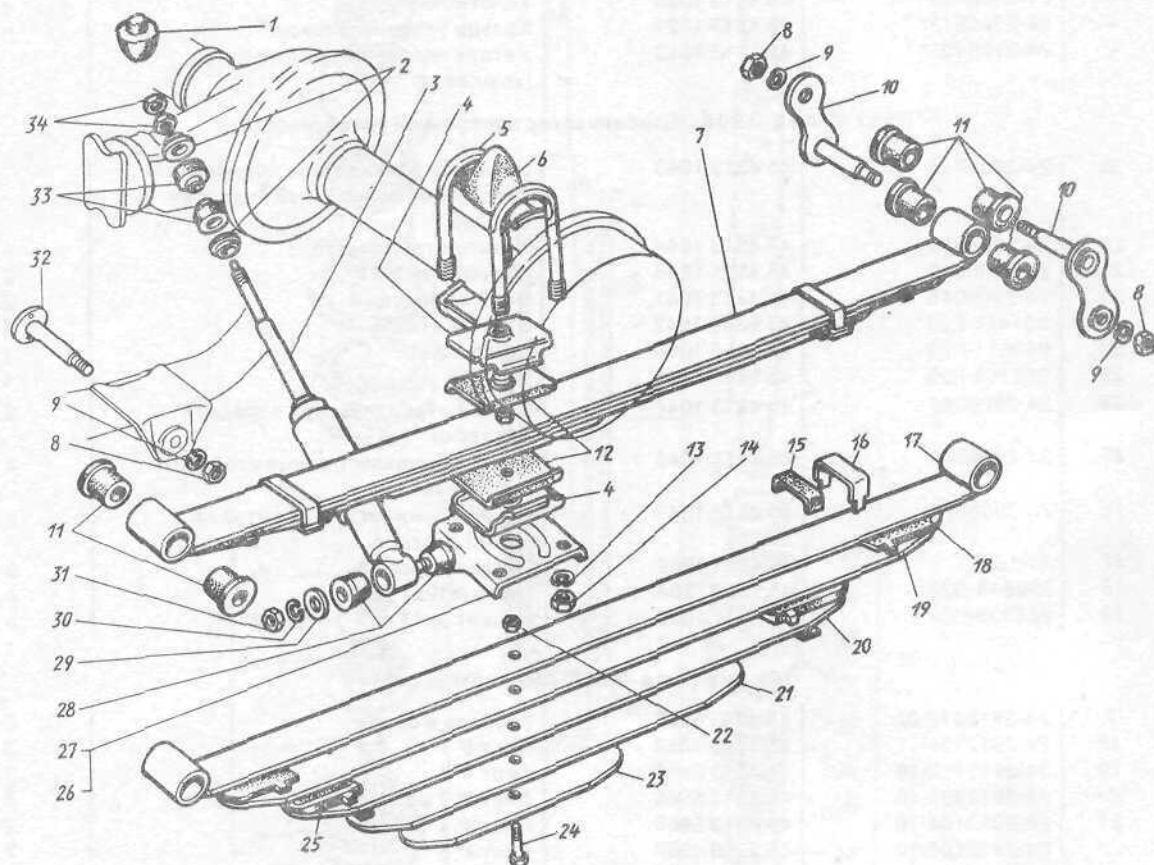
Рис. 35. Рессоры задние и крепление задних амортизаторов Примечание: Поз. 2, 3, 28...31, 33, 34 см. в подгруппе 2915.
