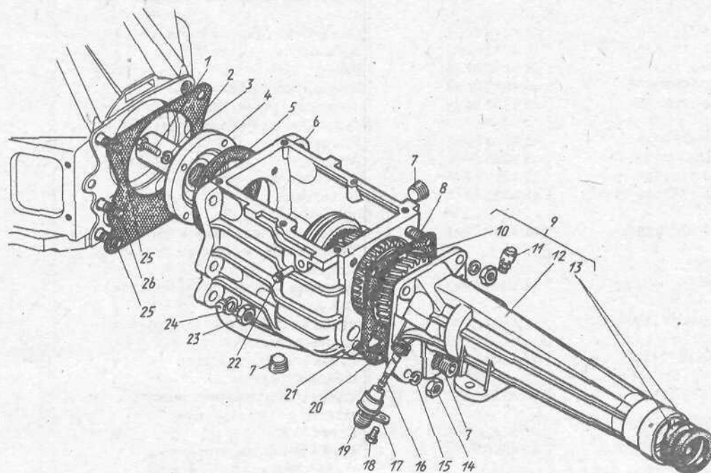
Рис. 25. Картер и удлинитель со вторичным валом коробки передач
