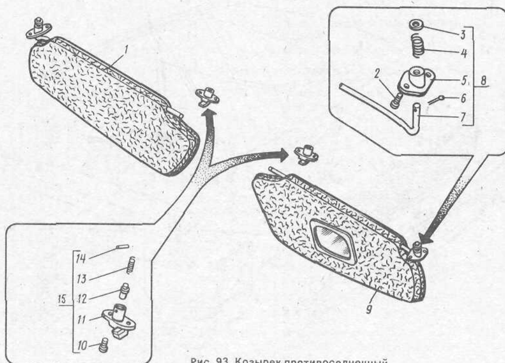
Рис. 93. Козырек противосолнечный
