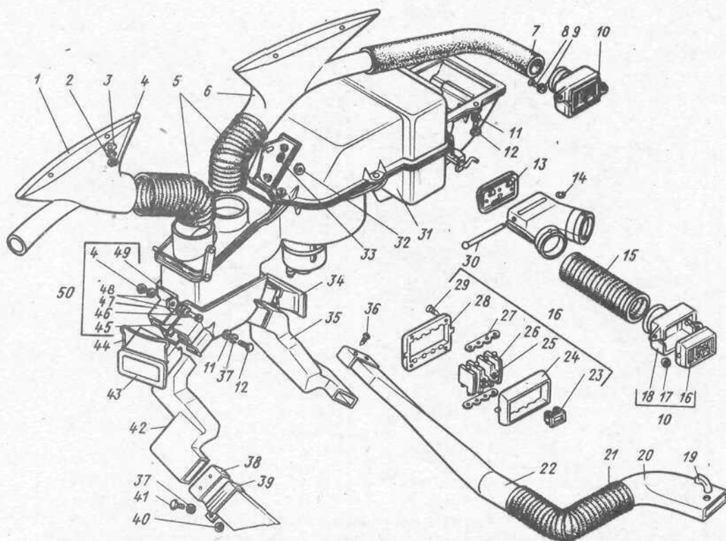
Рис. 89. Отопление и вентиляция
