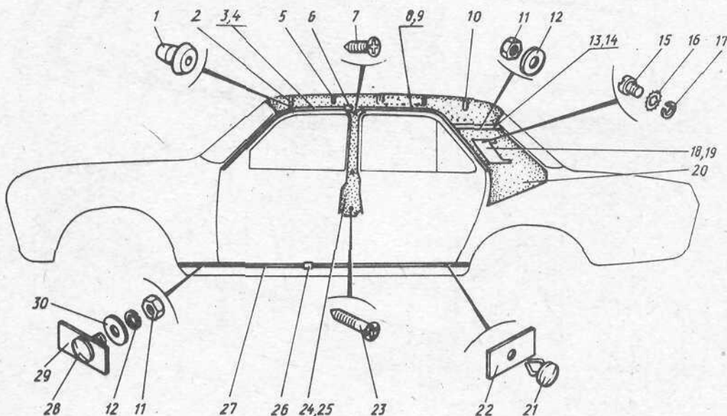
Рис. 76. Боковина, крыша, обивка крыши
