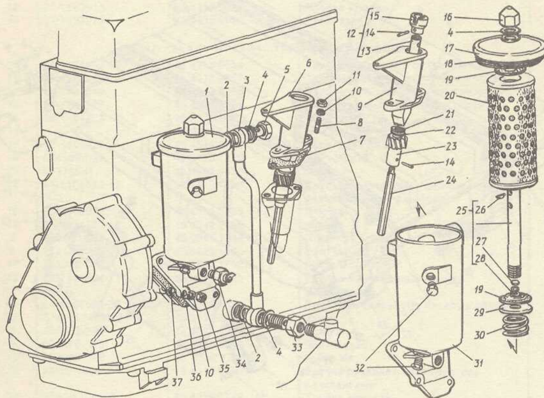
Рис. 9. Привод распределителя зажигания и фильтр очистки масла Примечание. Поз. 34 см. в подгруппе 3829
