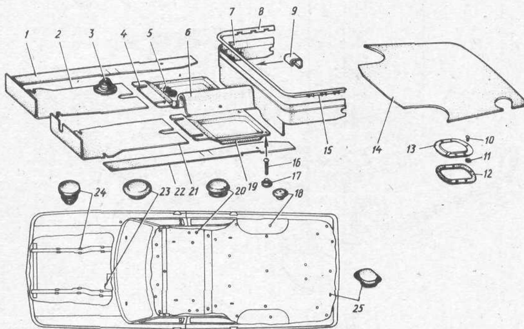
Рис. 70. Пол, кофух пола, коврики пола и багажника
