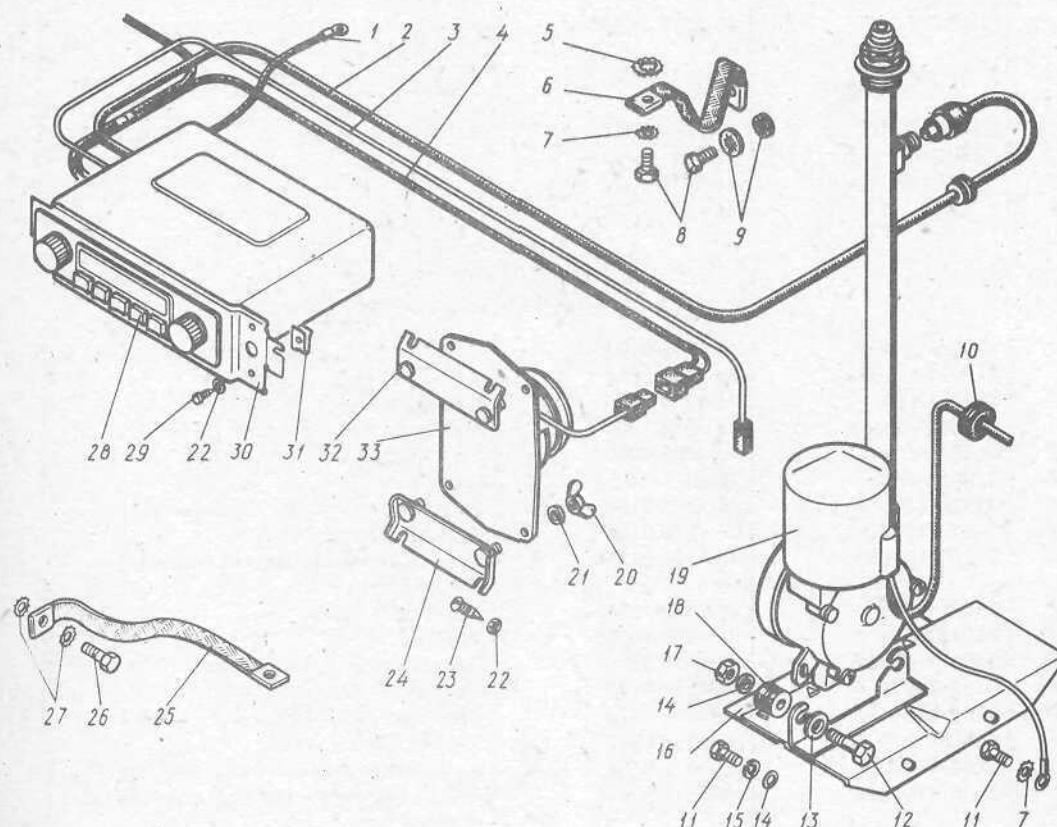
Рис. 87. Радиооборудование
