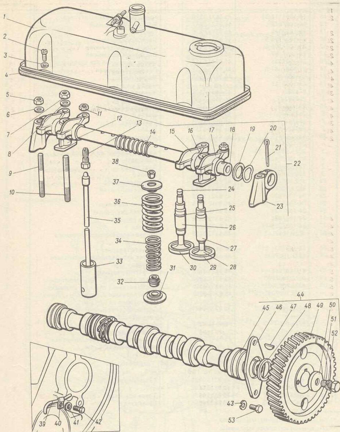
Рис. 5. Вал распределительный, клапаны и толкатели клапанов двигателя
