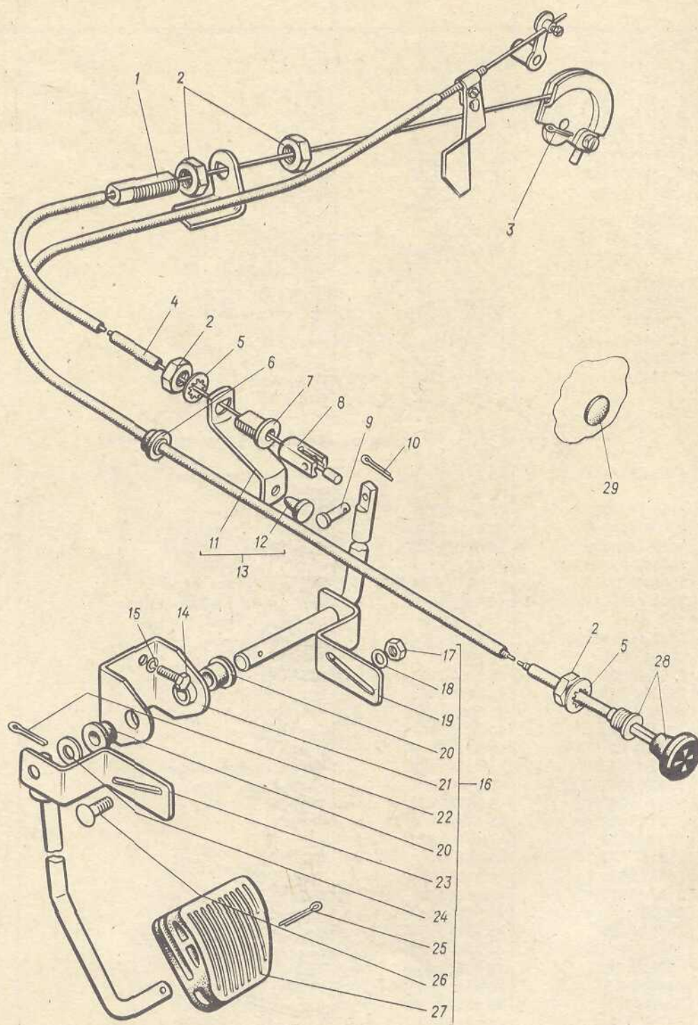
Рис. 15. Акселератор
