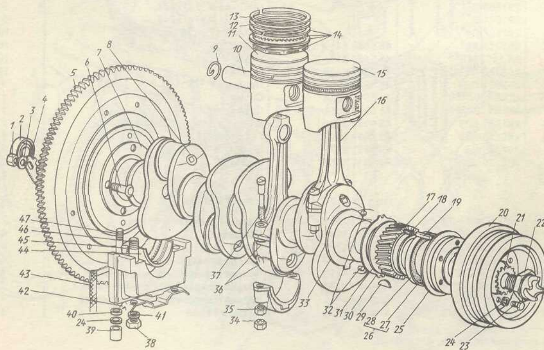
Рис. 4. Поршни, шатуны, вал коленчатый и маховик двигателя
