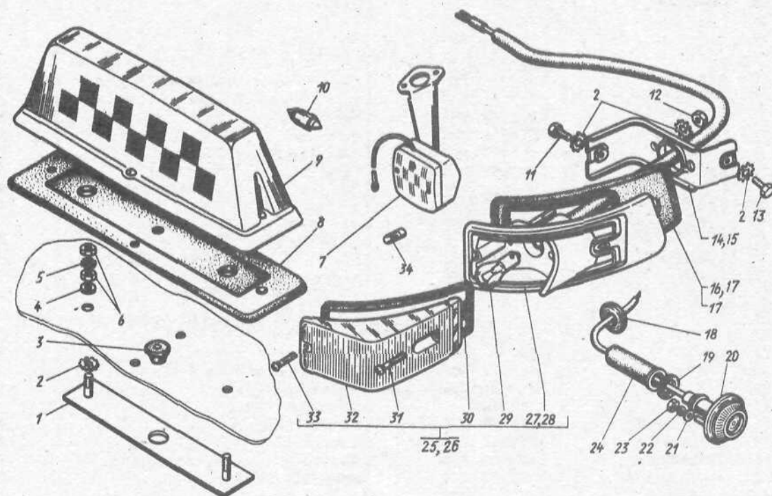
Рис. 65. Указатели поворота, повторители и опознавательные фонари такси Примечание. Поз. 1...6, 7, 8, 9, 10, 34 см в подгруппе 3757 (для модели ГАЗ-24-11).
