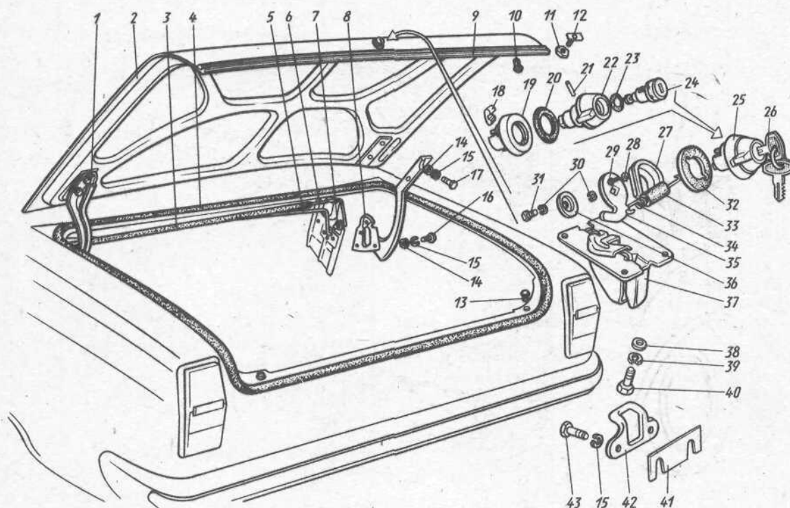
Рис. 78. Крышка багажника, петли, упор, замок крышки багажника.
