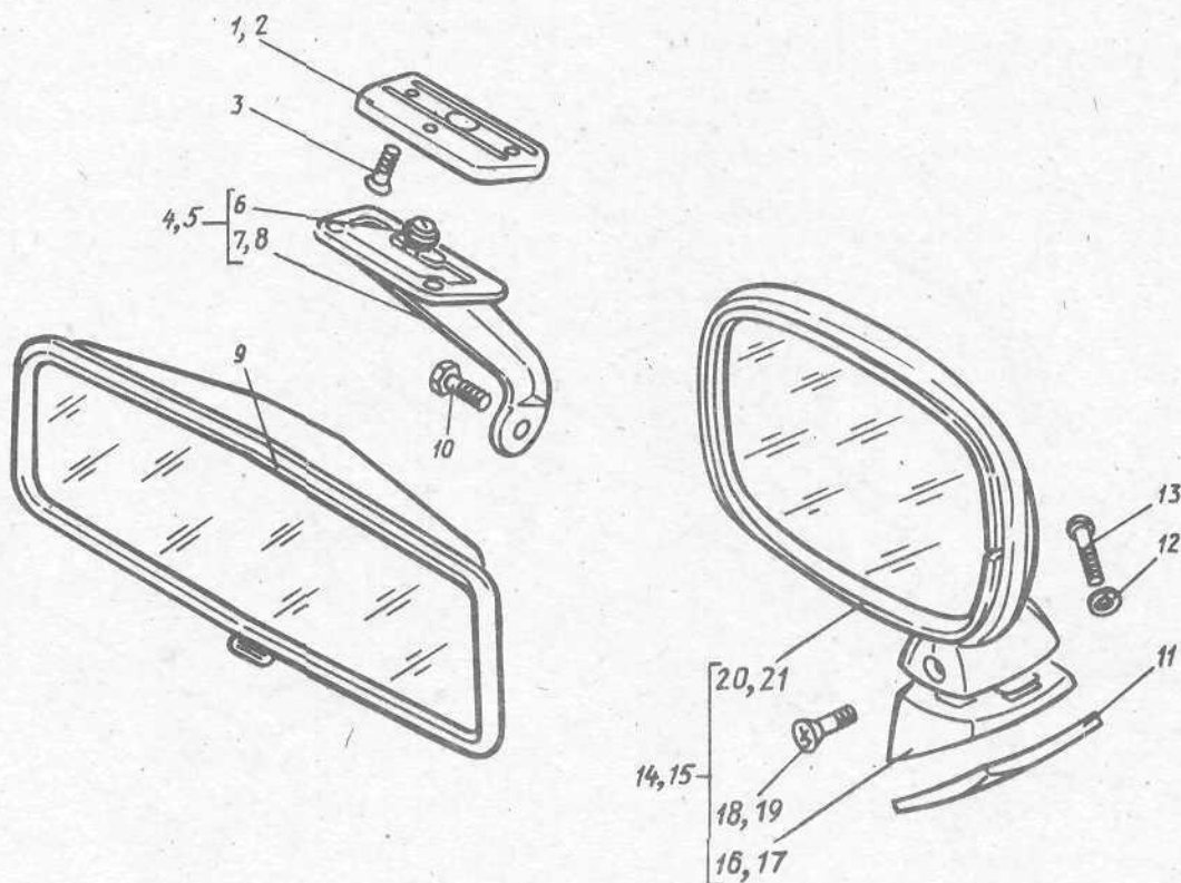
Рис. 91. Зеркала
