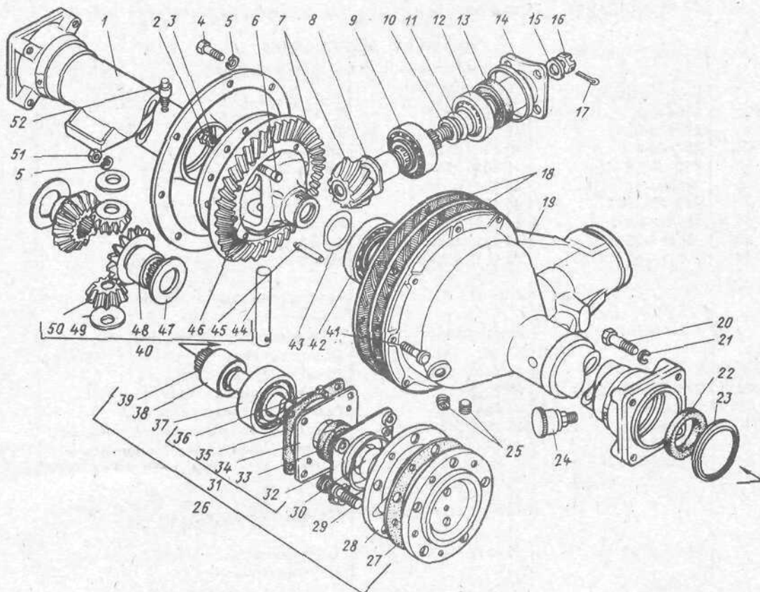
Рис. 28. Мост задний
