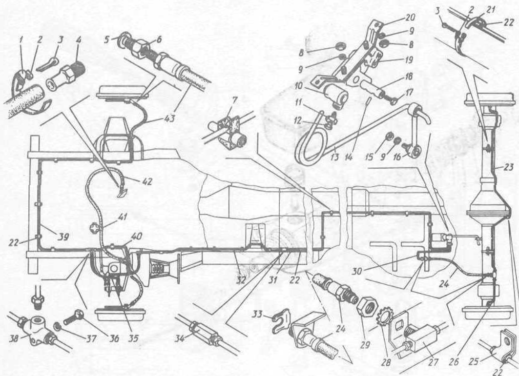
Рис. 49. Трубопроводы и регулятор тормозного момента гидравлических систем
