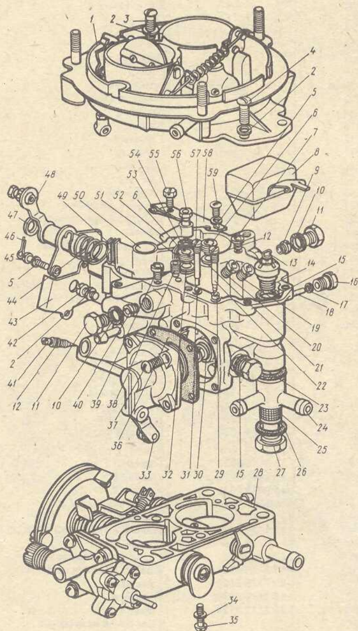
Рис. 14. Карбюратор
