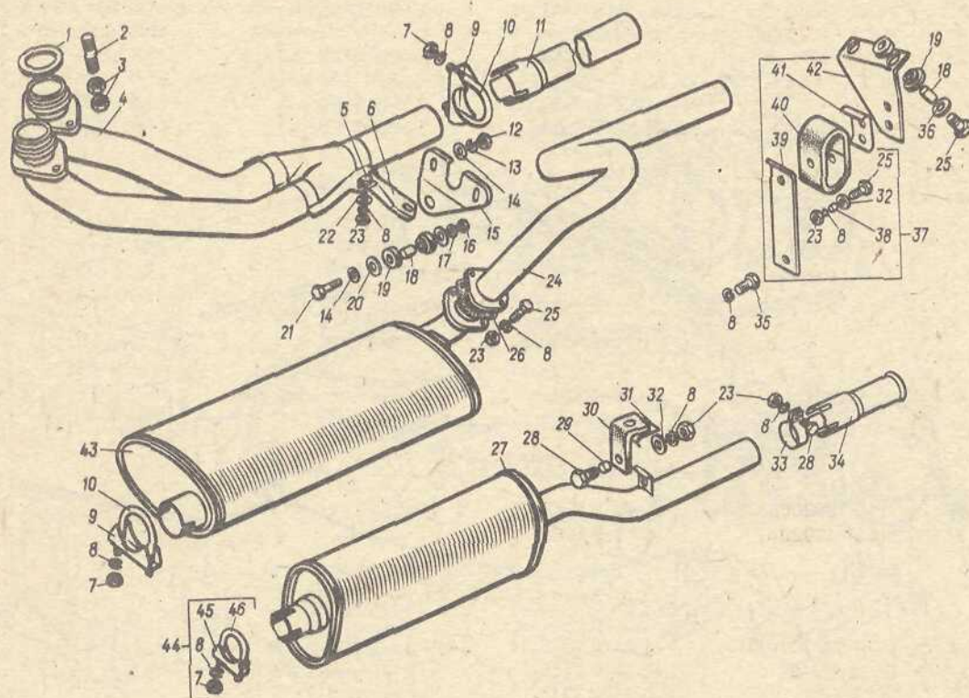
Рис. 17. Глушитель выхлопа и трубы выхлопные
